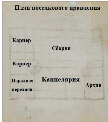
План поселкового правления. ОКВ. 1897 г. Масштаб: 2 аршина в дюйме. ГАОО. Ф. 37. Оп. 3. Д. 277. Л. 10
