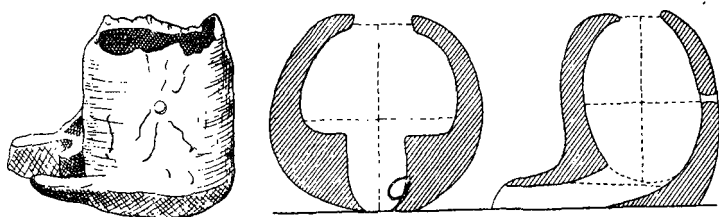
Рис. 9. Плавильная печь (из раскопок в Силезии)
