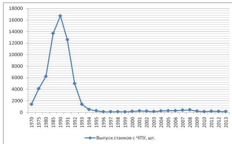
Рис. 3. Выпуск станков с ЧПУ в РФ (1970—2013) [14]
