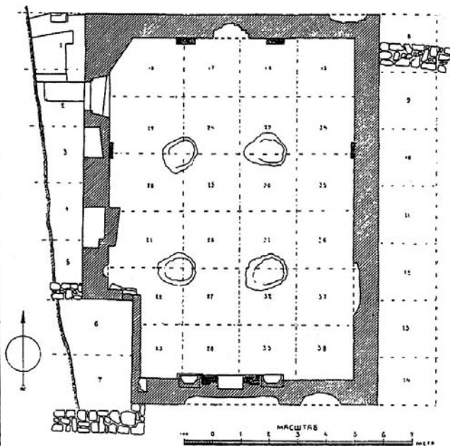
Рис. 11. План развалин мечети в Чуфут-Кале по раскопкам 1928–29 гг. [Боданинский, Засыпкин, 1929, рис.2]
