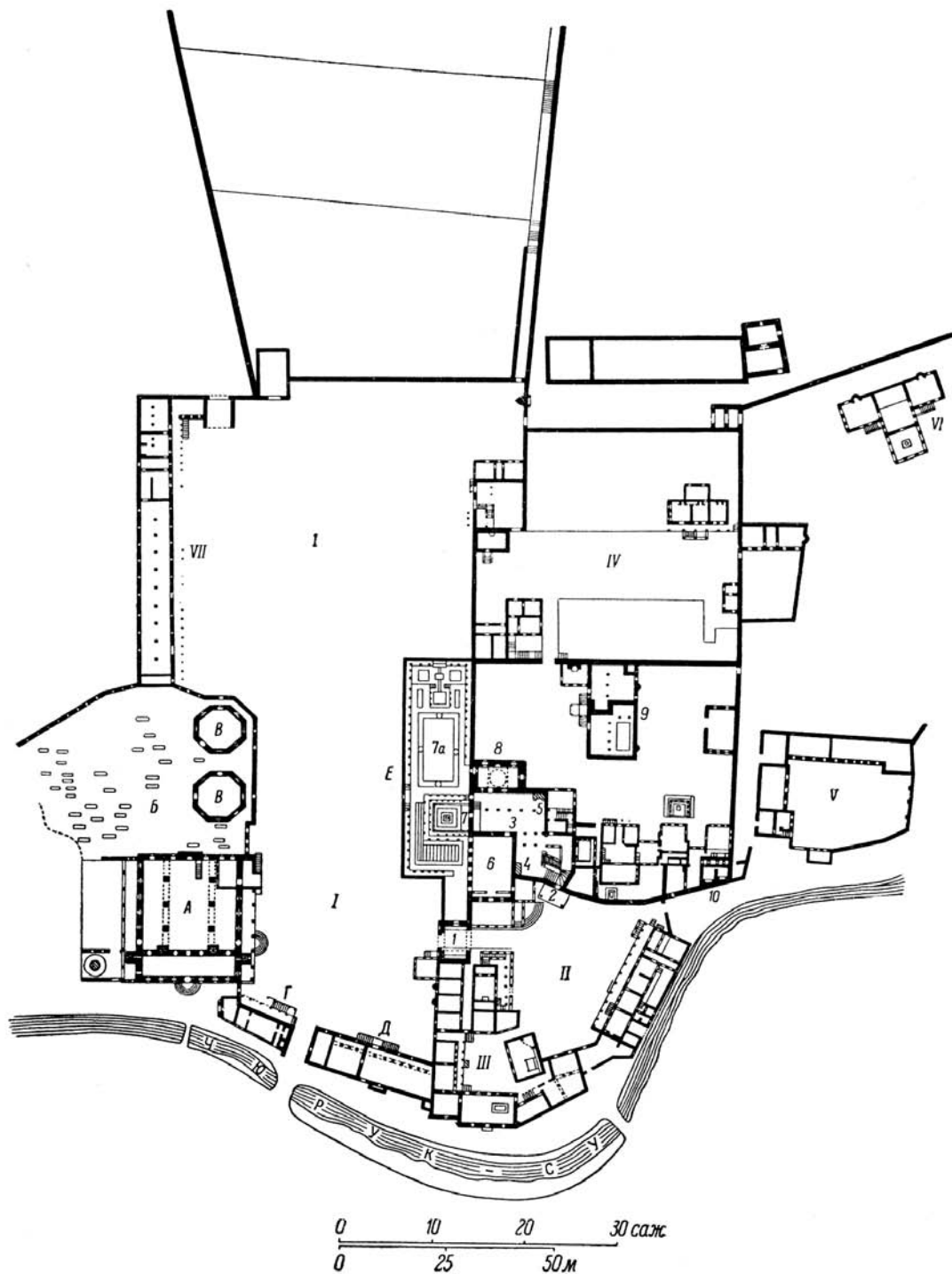
Рис. 23. План ханского дворца в Бахчисарае, составлен В.Гести в 1798 г.: I – большой двор; II – внутренний двор (Посольский); III – кухонный двор; IV – задний двор; V – пекарский двор; VI – старый дворец; VII – конюшня. А – мечеть 1740 г.; Б – ханское кладбище; В – дюрбе ханского кладбища; Г – свитский корпус; Д – комнаты для гостей; Е – главный корпус. 1 – ворота; 2 – «железные ворота», 1503 г.; 3 – фонтанный дворик; 4 – «фонтан слез», 1763 г.; 5 – «Золотой фонтан», 1733 г.; 6 – Диван (зал Совета и Суда); 7 – Золотой, или фруктовый, кабинет, 1764 г.; 7а – цветник с фонтаном и бассейном; 8 – мечеть 1741 г.; 9 – гарем; 10 – баня [Якобсон, 1964, рис.47]
