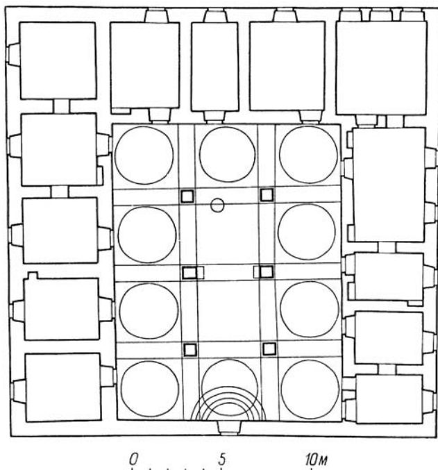
Рис. 21. Медресе Менгли Гирей-хана («Зинджирлы-медресе») в Эски Салачик [Якобсон, 1964, рис.46]
