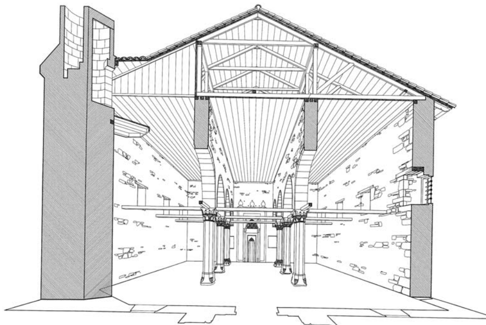
Рис. 7. Реконструкция внутреннего пространства т.н. мечети Узбека в Эски-Кырым (совр. г. Старый Крым). Второй строительный период [Кирилко, 2008б, рис.46]
