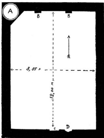
Рис. 10. План развалин мечети в Чуфут-Кале [Акчокраклы, 1928, рис.9]
