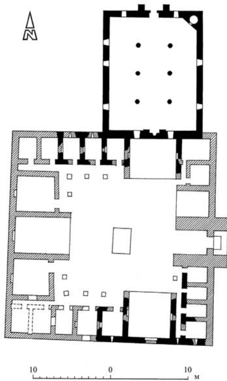
Рис. 1. План медресе и т.н. мечети Узбека в Эски-Кырым (совр. г. Старый Крым). Сплошной заливкой обозначены стены строений, сохранившиеся на всю высоту, штриховкой – нижние части кладок [Кирилко, 2008б, рис.1]
