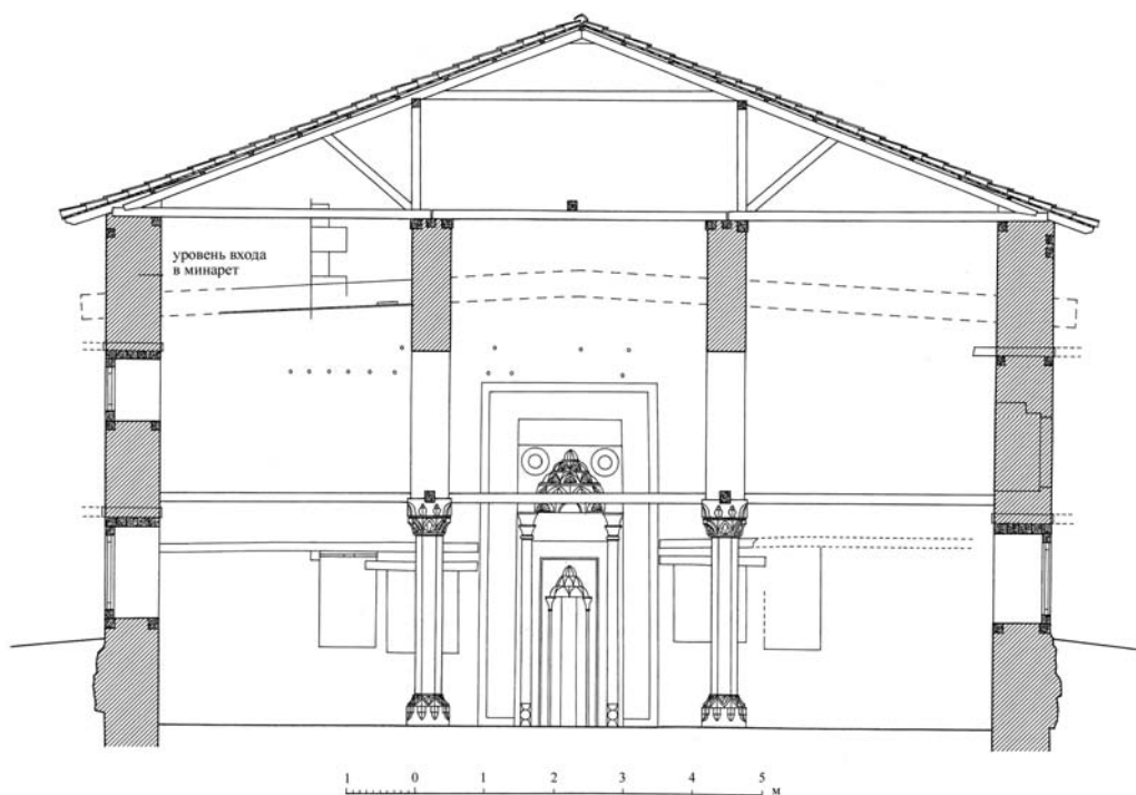
Рис. 6. Поперечный разрез т.н. мечети Узбека в Эски-Кырым (совр. г. Старый Крым). Вид с севера [Кирилко, 2008б, рис.18]
