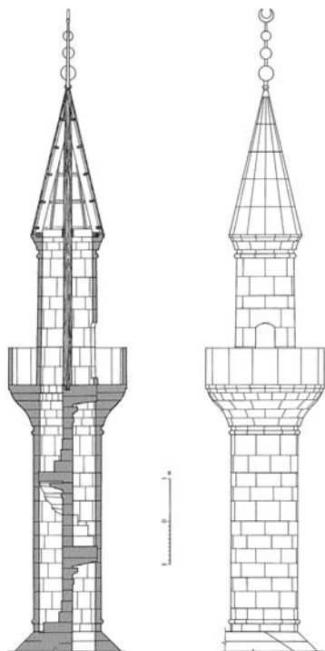
Рис. 5. Реконструкция минарета т.н. мечети Узбека в Эски-Кырым (совр. г. Старый Крым): 1 – разрез по оси С-Ю, 2 – южный фасад [Кирилко, 2008б, рис.29]
