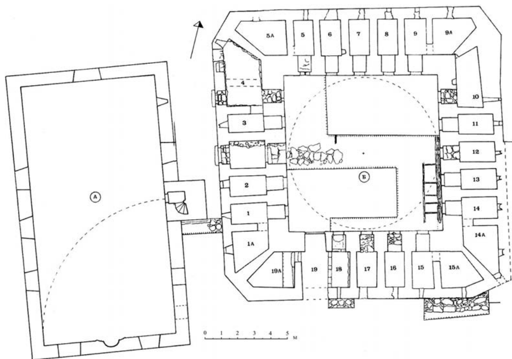
Рис. 18. План мечети Шукурла-эфенди и текке в Гёзлëвë [Кутайсов, Кутайсова, 2007, с.96]
