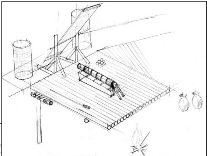
Кяриз-тайник и артиллерийский роскат казанской крепости середины XVI в. Реконструкция А.Н.Хабибуллина
