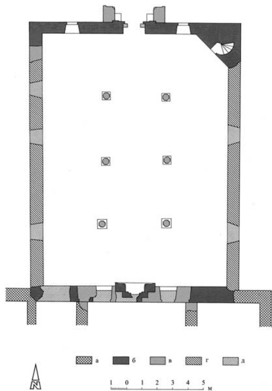
Рис. 2. План т.н. мечети Узбека в Эски-Кырым (совр. г. Старый Крым). Картограмма строительных периодов. Условные обозначения кладок: а – медресе, б – первого строительного периода, в – второго строительного периода, г – третьего строительного периода, д – современных ремонтных дополнений [Кирилко, 2008б, рис.14]
