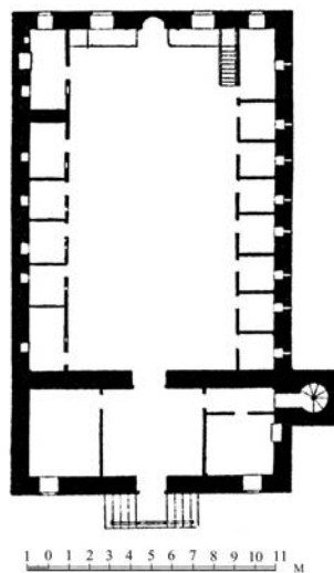
Рис. 13. План мечети Текие-Хан-Джами в Карасу-Базаре [Засыпкин, 1927, рис.12]
