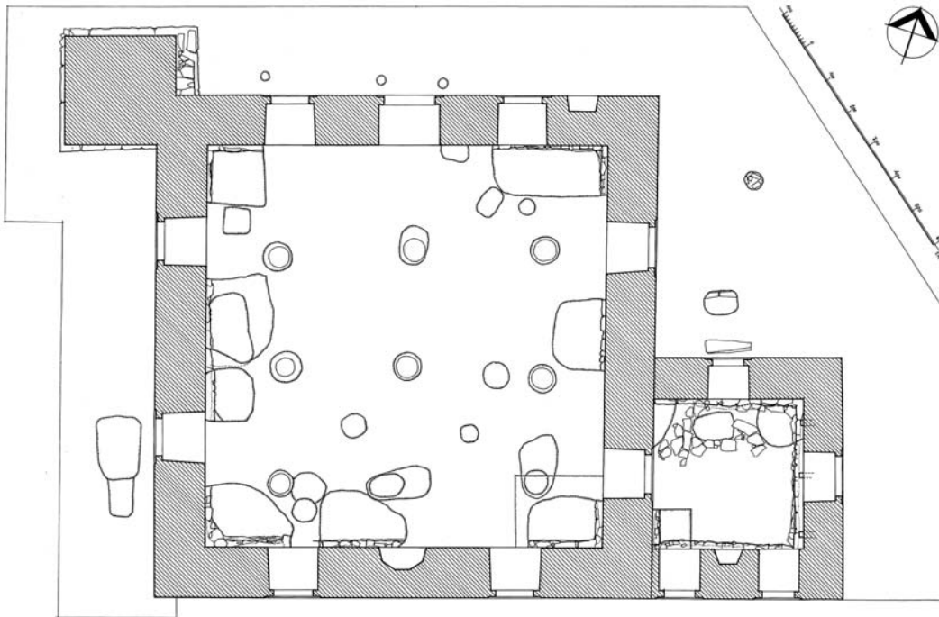
Рис. 16. План мечети в Эски-Сарае по результатам раскопок 1991 г. Чертеж В.П.Кирилко
