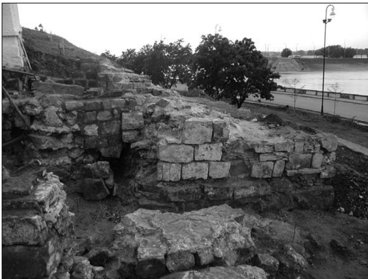
«Северная» башня татарской крепости первой половины XVI в. (реконструкция плана по археологическим данным, фотография с археологических раскопок, реконструкция башни А.Н.Хабибуллина)
