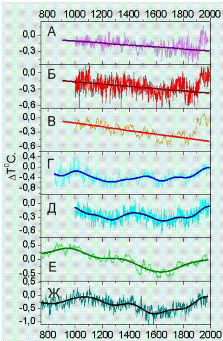
Рис. 1. Палеореконструкции температуры Северного полушария Земли: А – NHM (Mann et al., 1999); Б – NHJ (Jones et al., 1998); В – NHC (Crowley and Lowery, 2000); Г – NHE (Esper et al., 2002); Д – NHV (Briffa, 2000); Е – NHL (Loehle, 2007); Ж – NHMb (Moberg et al., 2005).
