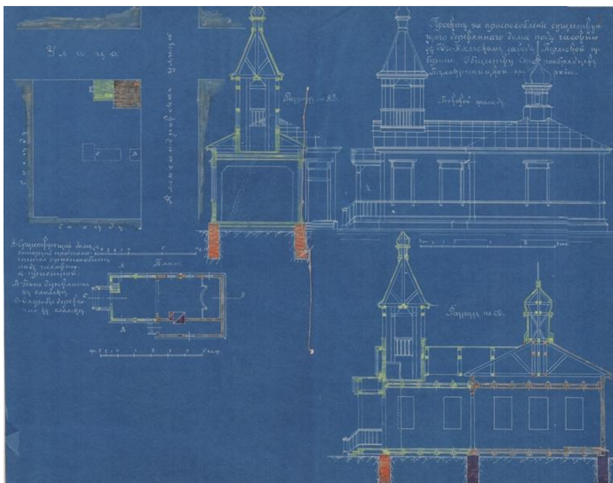
Проект на приспособление существующего деревянного дома под старообрядческую часовню в Юго-Камском заводе Пермского уезда. 1917 г.
