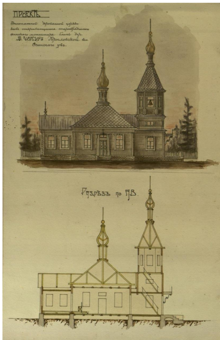
Проект деревянной церкви вновь открывающегося старообрядческого женского монастыря близ д. Верхний Чекур Крыловской волости Осинского уезда. 1917 г. ГАПК. Ф. 36. Оп. 5. Д. 82. Л. 2об.
