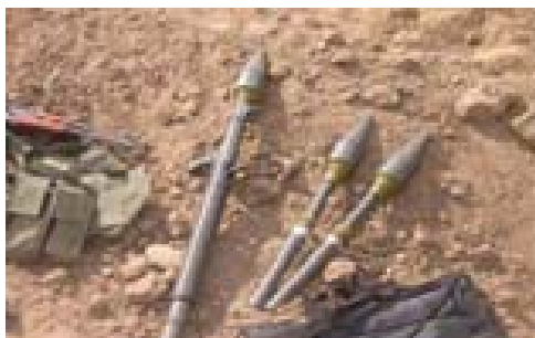
Ракеты "Аль-Ясин" производства Хамас. Максимальная дальность: около 250 м. Приблизительная бронепробиваемость: до 200 мм (сталь).
