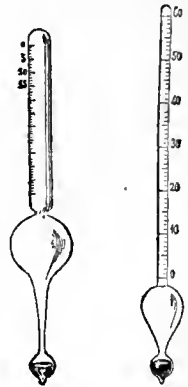
FIG. 2. Salimeter.
