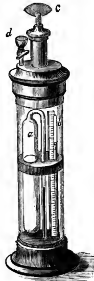
FIG. 1.—Oersted's Apparatus.
