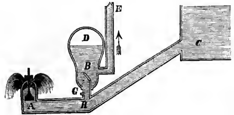
FIG. 1.—Hydraulic Ram.
