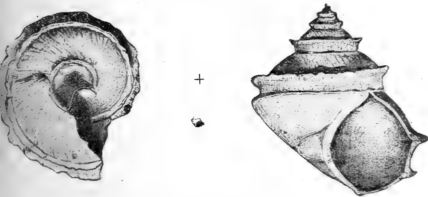
La figura in mezzo è in grandezza naturale. Le due figure laterali mostrano la conchiglia ingrandita.
