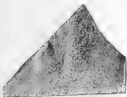
Fig. 2. — Nevrodontopteris auriculata sotto Pic Ciadin presso al ric. Marinelli.
