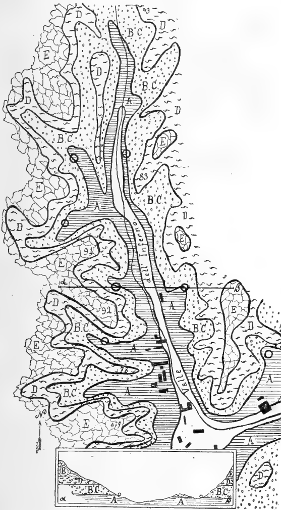
Fig. IV. a — Carta geologica della Valle dell'Inferno, presso Roma, con una sezione corrispondente ad \alpha - \beta . Scala delle lunghezze 1:22500 e dell'altezze (sezione) 1:4500. I circoletti, tanto in questa figura come nelle seguenti, indicano sempre le sorgenti; le lettere ed i segni corrispondono sempre alle stesse rocce, come fu avvertito nella spiegazione della Figura II. a , e cioè: A = Marne marine; B, C = Sabbie e Ghiaie (riunite nella figura per chiarezza); D = Sabbioni di duna; E = Tufi vulcanici.
