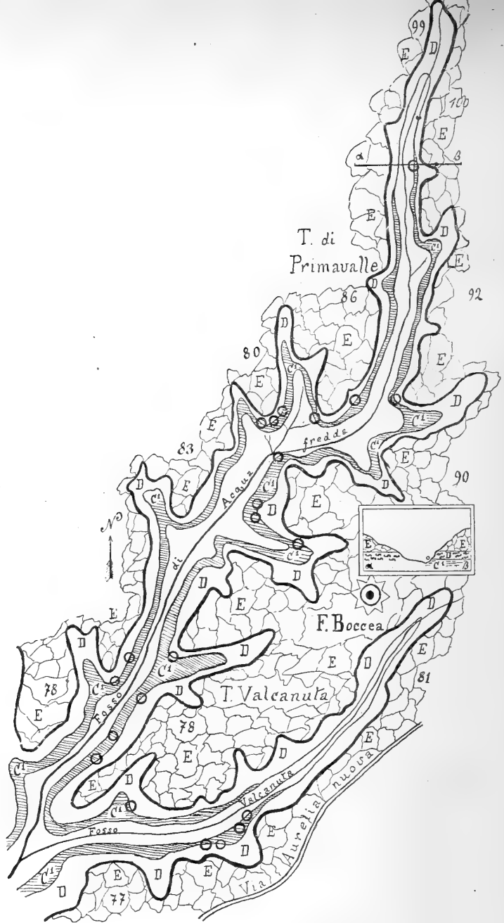
Fig. VI. a — Carta geologica della Valle del Fosso Acquafredda, con una sezione corrispondente alla linea α-β. Scala delle lunghezze 1:22500, delle altezze (sezione) 1:4500. I circoletti indicano le sorgenti; le lettere ed i segni rappresentano le formazioni solite e cioè: C 1 = Marne di stagno; D = Sabbioni di duna (senza segni per chiarezza); E = Tufi vulcanici.
