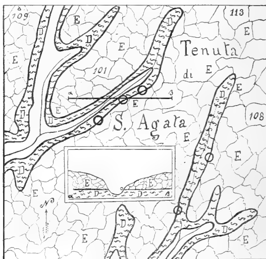
Fig. VIII. a — Carta geologica della Tenuta di S. Agata, con una sezione corrispondente alla linea \alpha - \beta . Scala delle lunghezze 1:20000 e delle altezze (sezione) 1:4000. I circoletti indicano le sorgenti. Le lettere ed i segni rappresentano le solite formazioni, e cioè: D = Sabbioni di duna; E = Tufi vulcanici.
