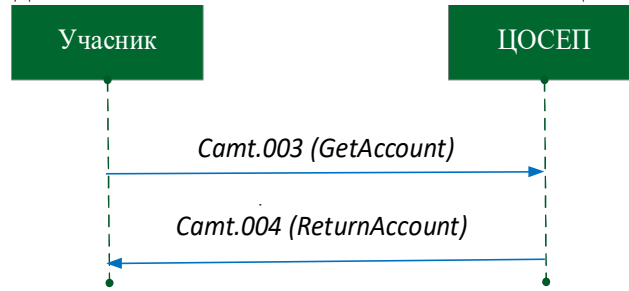
Рис. 1. Схема обміну повідомленнями camt.003 і camt.004 в pull-mode
