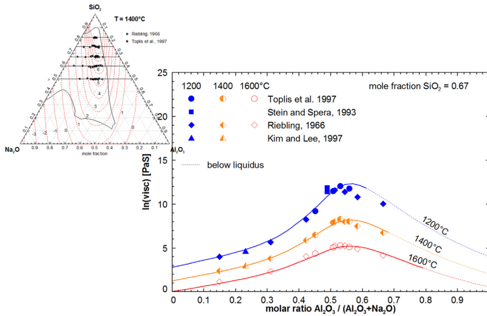
Fig. 19. Viscosity module – viscosities in \text{Na}_2\text{O}-\text{Al}_2\text{O}_3-\text{SiO}_2 .
