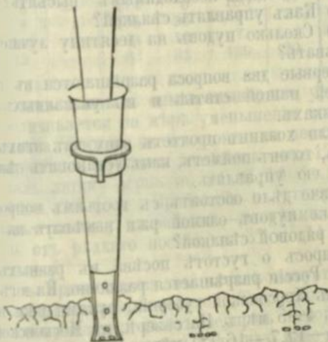
Рис. 6. Сошникъ Эльворти (видъ сзади).
