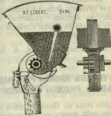
Рис. 5. Выбрасывающій приборъ (въ разрѣзѣ) сѣялки Энкерта „Новь—Миранда“.
