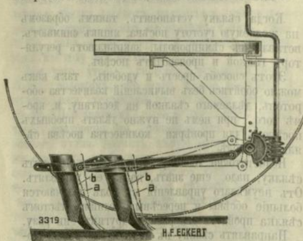
Рис. 9. Регуляторъ глубины сѣлки Энкерта.
