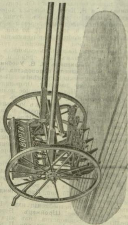
Рис. 4. 7-рядная сѣлка Эльворти.
