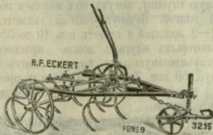
Рис. 3. 9-тизубной культиваторъ Энкерта „Коршунъ“ съ колесомъ.
