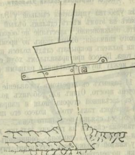
Рис. 7. Сошникъ Эльворти (видъ съ боку).
