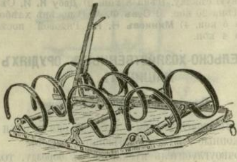
Рис. 2. Пружинная борона американской системы. Со склада Т-ва „Работник“.
