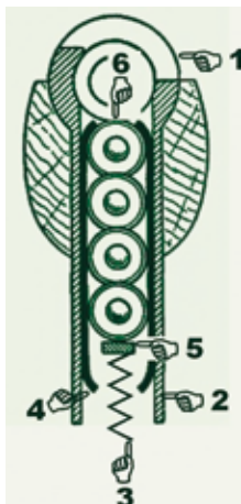
Система подачи патронов Манлихера: 1 – патронник 2 – стенка магазина 3 – пружина подавателя 4 – стенка пачки 5 – подаватель 6 – патрон
