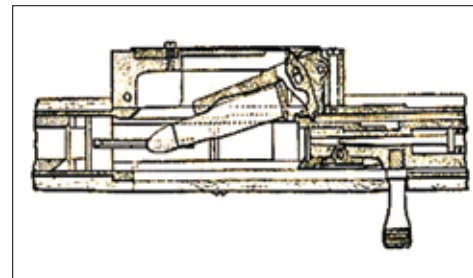
Система подачи патронов Манлихера: 1 – патронник 2 – стенка магазина 3 – пружина подавателя 4 – стенка пачки 5 – подаватель 6 – патрон
