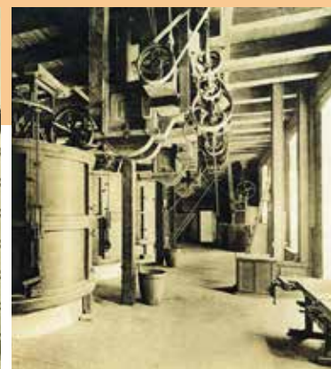
Foto: www.zacherfabrik.at
