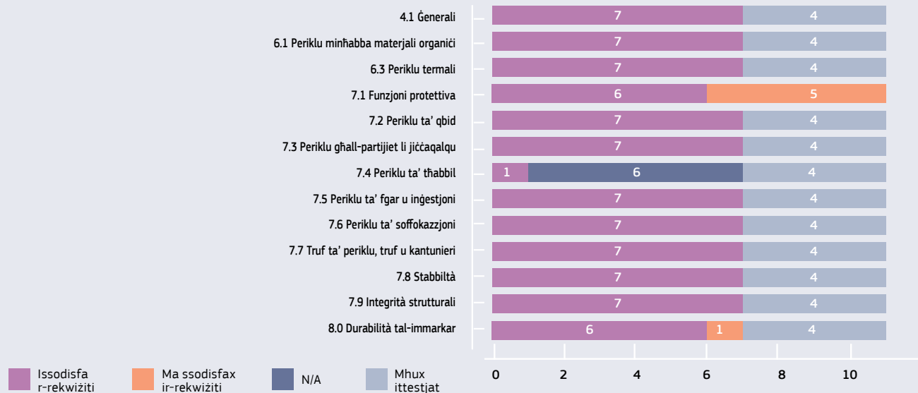
Figure 5 - Riżultati tat-test għal kull klawżola ta' EN 1466:2014 (N=11)
