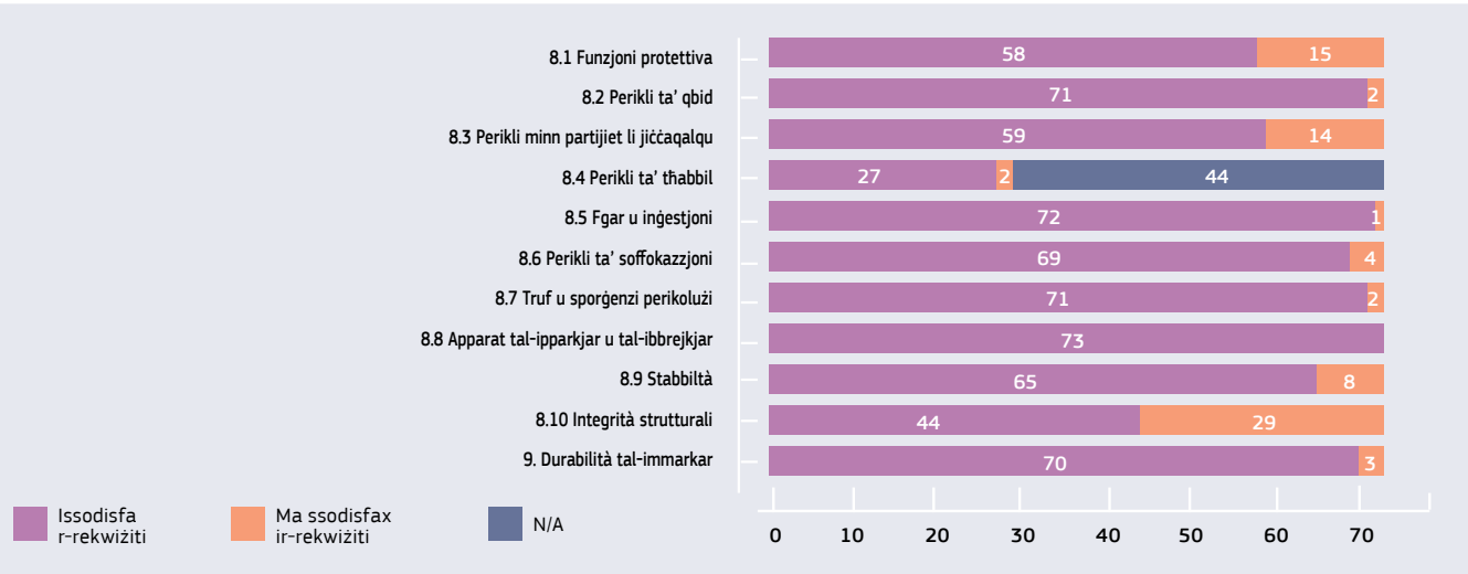
Figura 4 - Rizultati tat-test għal kull klawżola ta' EN 1888-1:2018 (N=73)
