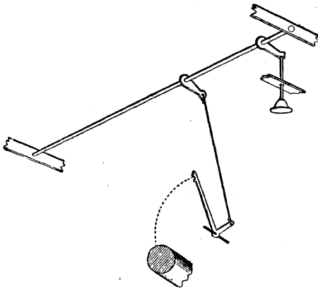
Рис. 3. Смиль-Премьеръ. Механизмъ буквенныхъ стержней.
