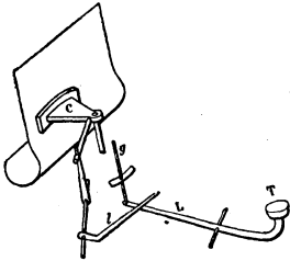
Рис. 9. Гаммонд. Схема функционирования печатающего механизма.
