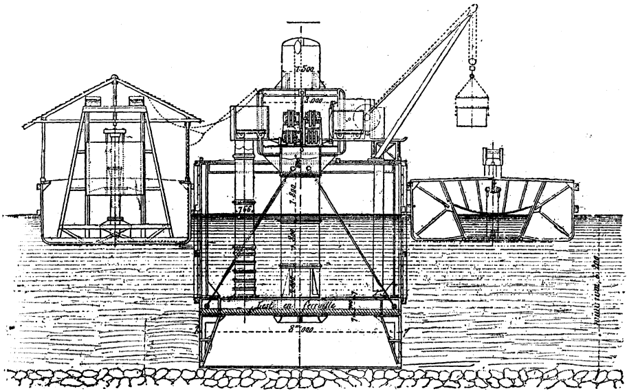
Рис. 3. Поперечный разръзъ воздушнаго колокола въ Pointe des Galets.
