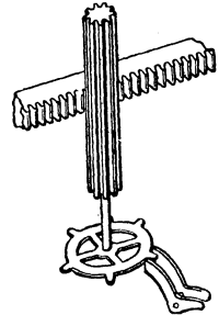
Рис. 1. Якорный спускъ.
