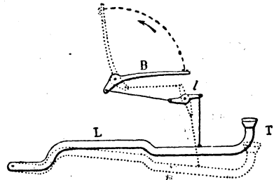
Рис. 7. Ремингтонъ. Механизмъ клавиши и печатнаго стержня.
