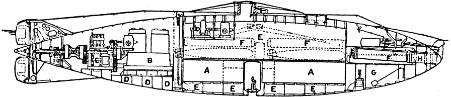
Рис. 3. Разрѣзъ сѣверо-американской подводной лодки «Adder». А—аккумуляторныя батареи; В—газовый двигатель; С—динамомашина; D—водонепроницаемые отдѣленія; E—балластные цистерны; F—резервуары для сжатого воздуха; G—газолиновая цистерна; H—минная пушка.
