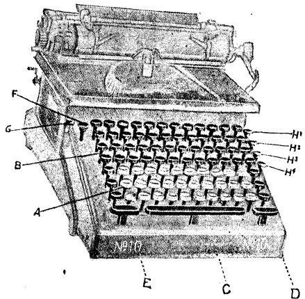
Рис. 12. Смисъ-Премьеръ № 10. Полная клавиатура.
