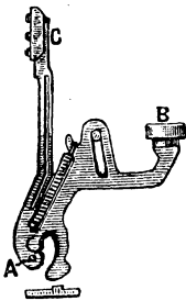
Рис. 4. Типо. Нормальное положеніе клавиши.
