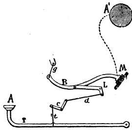
Рис. 10. Юст (новая модель). Схема печатанія.
