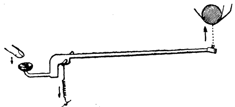
Рис. 2. Геральдъ. Механизмъ печатанія.
