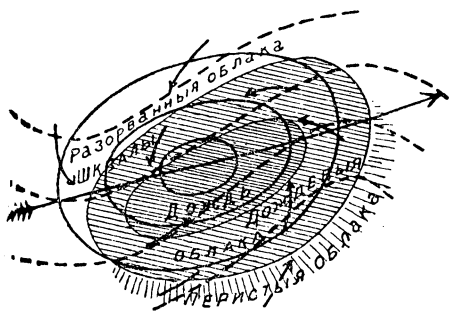
— ИЗОБАРЫ --- ИЗОТЕРМЫ
