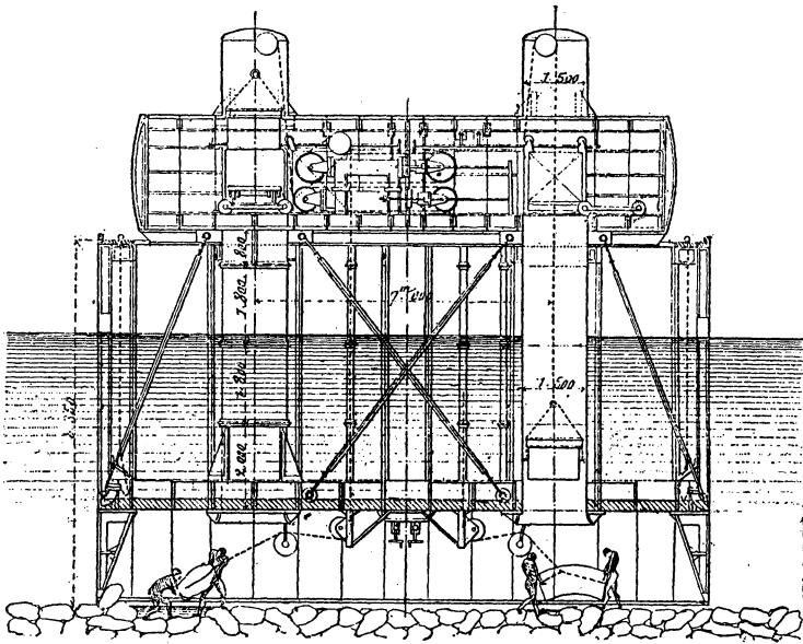
Рис. 4. Продольный разръзъ воздушнаго колокола въ Pointe des Galets.
