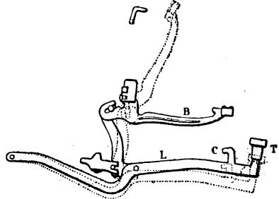
Рис. 6. Ундервудъ. Схема функционирования буквенныхъ стержней.
