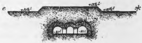
Профиль по линіи е ж.
