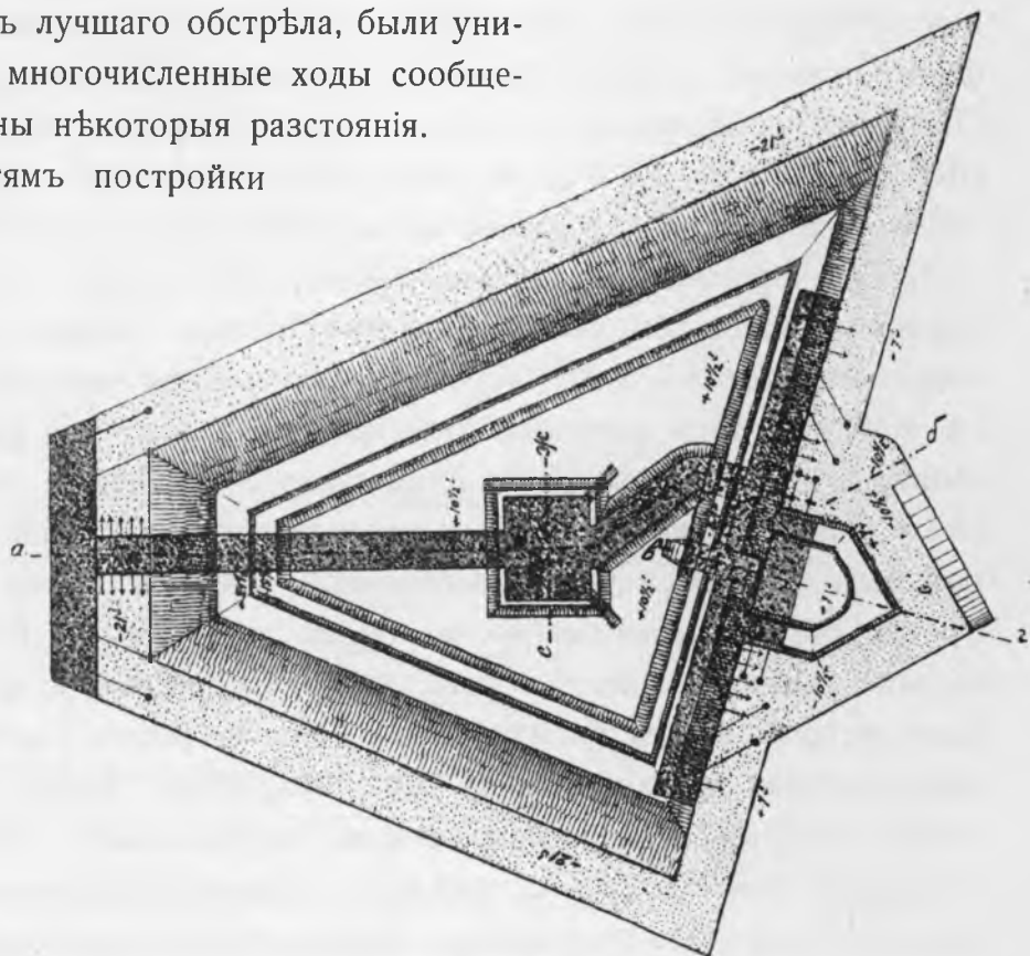
Укрѣпленіе № 3.
