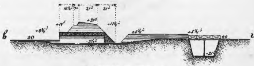
Профиль по линіи в г.
