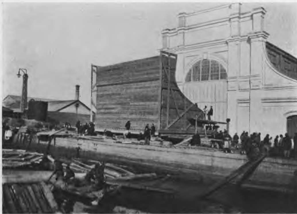
Готовый кессонъ на берегу въ Портъ-Аргурѣ.
