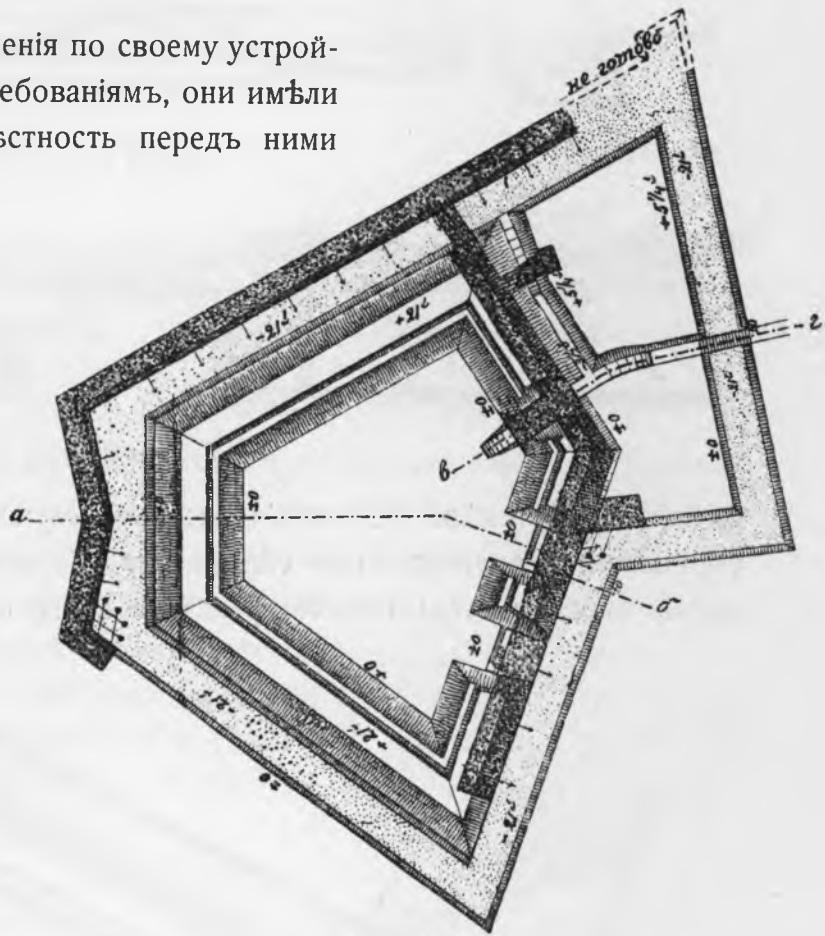
Фортъ № 2.
