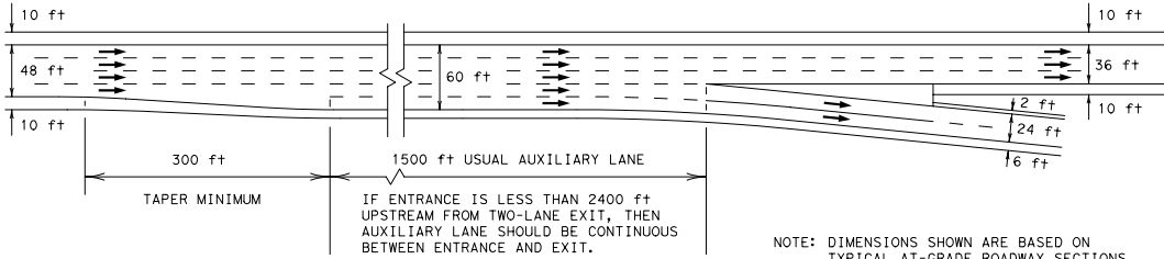
MULTILANE DIVERGE
