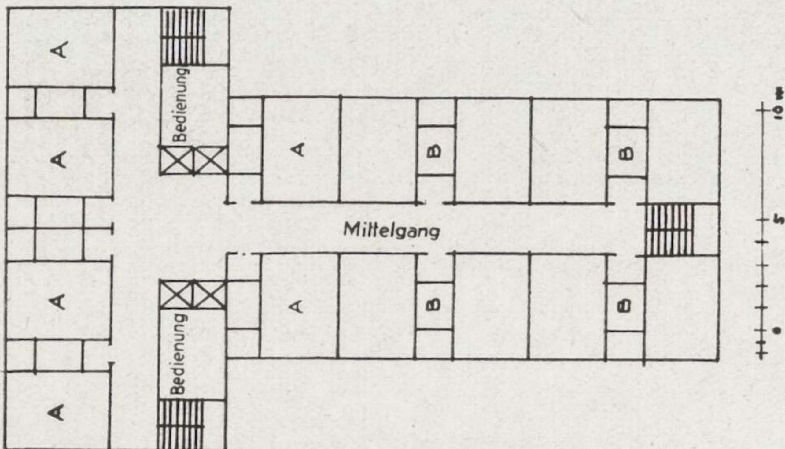
anordnungsschema der 1 und 2 zimmerwohnungen
