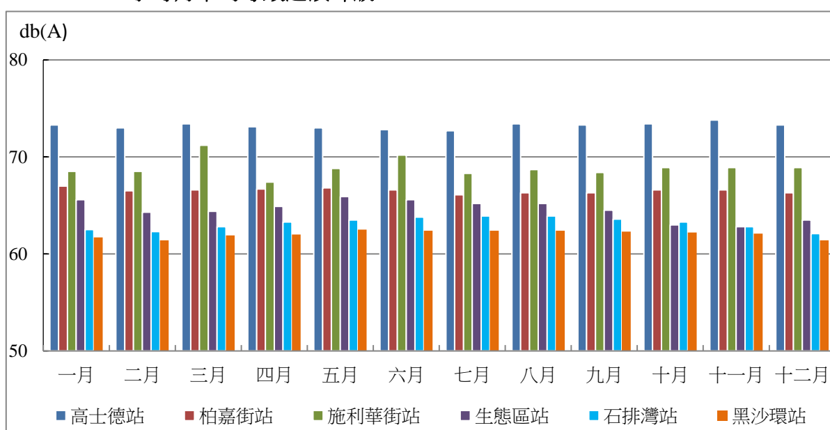
圖 3.1 2019 年各環境噪聲監測站 24 小時月平均等效連續聲級 ( L_{eq} ) 變化圖
