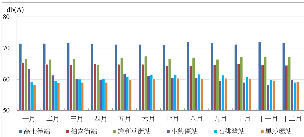
圖 3.3 2019 年各環境噪聲監測站夜間月平均等效連續聲級（ L_{eq} ）變化圖
