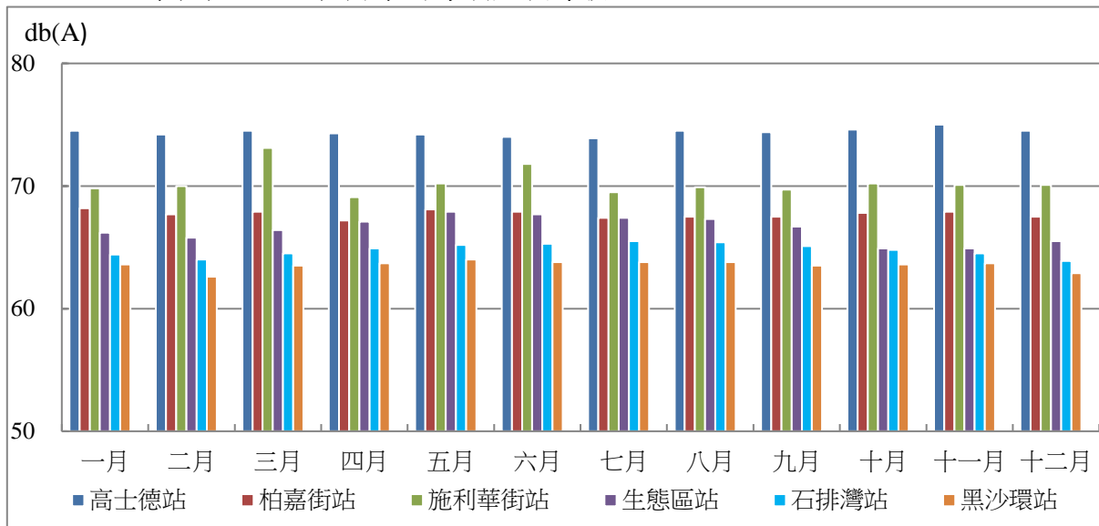
圖 3.2 2019 年各環境噪聲監測站日間月平均等效連續聲級（ L_{eq} ）變化圖
