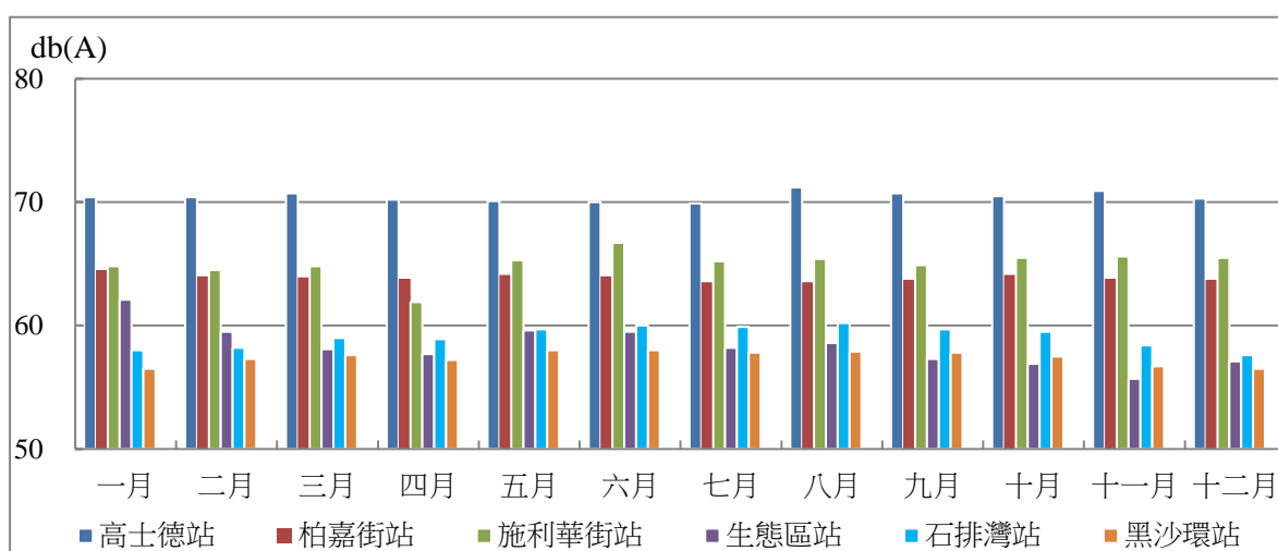
圖 3.5 2019 年各環境噪聲監測站深宵月平均等效連續聲級 ( L_{eq} ) 變化圖
