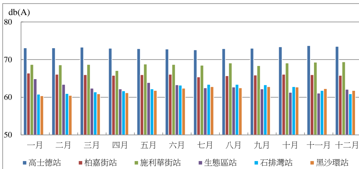
圖 3.4 2019 年各環境噪聲監測站黃昏月平均等效連續聲級 ( L_{eq} ) 變化圖
