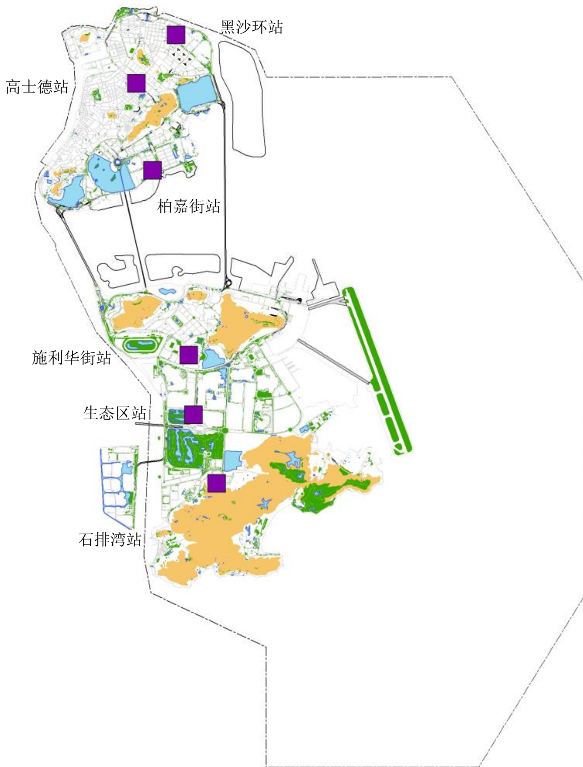
图 1.1 环境噪声监测站位置
