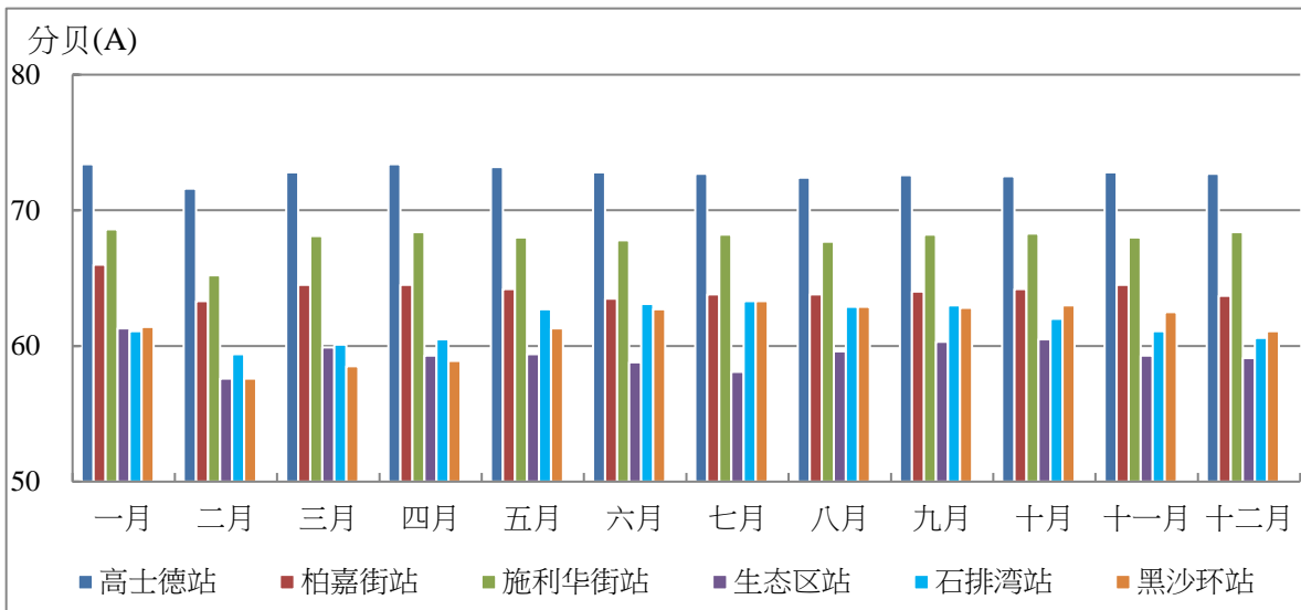
图 3.4 2020 年各环境噪声监测站黄昏月平均等效连续声级 (Leq) 变化图
