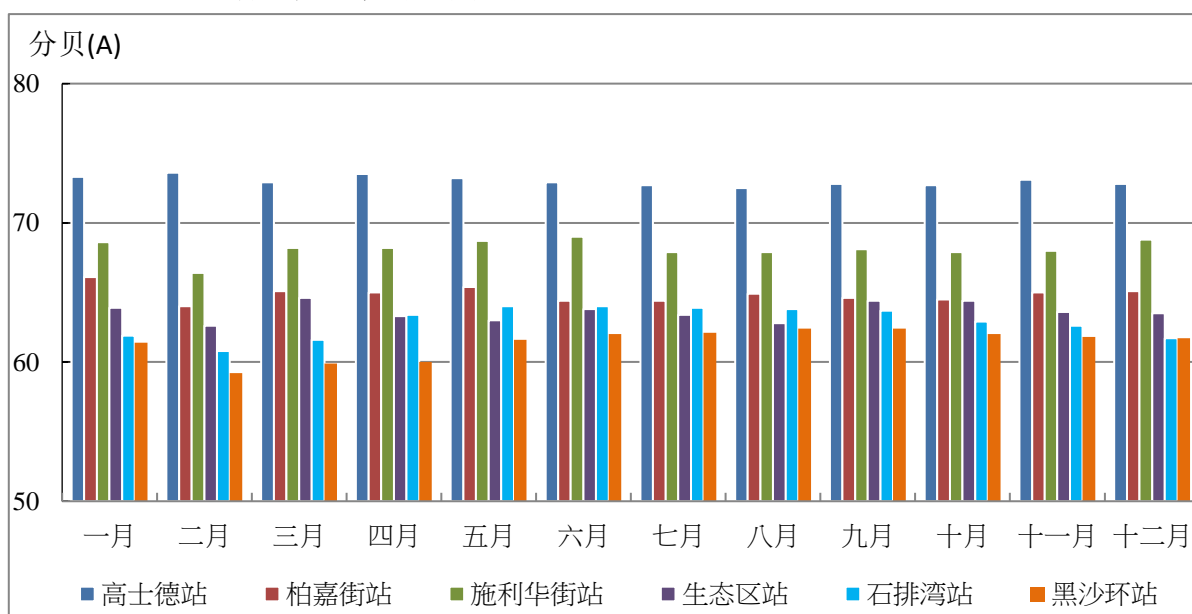
图 3.1 2020 年各环境噪声监测站 24 小时月平均等效连续声级 ( L_{eq} ) 变化图
