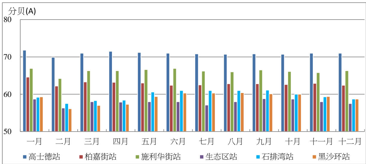
图 3.3 2020 年各环境噪声监测站夜间月平均等效连续声级 (Leq) 变化图
