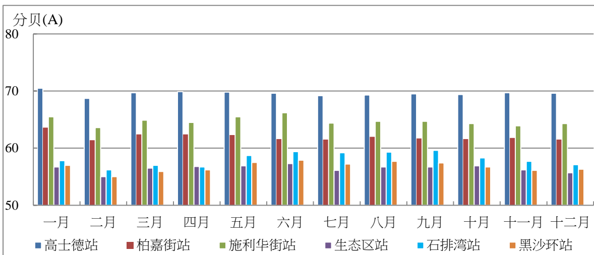
图 3.5 2020 年各环境噪声监测站深宵月平均等效连续声级 (Leq) 变化图
