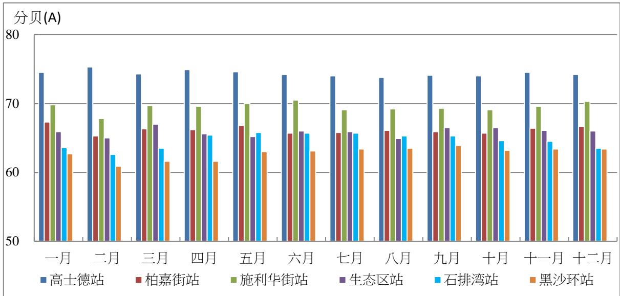
图 3.2 2020 年各环境噪声监测站日间月平均等效连续声级 (Leq) 变化图
