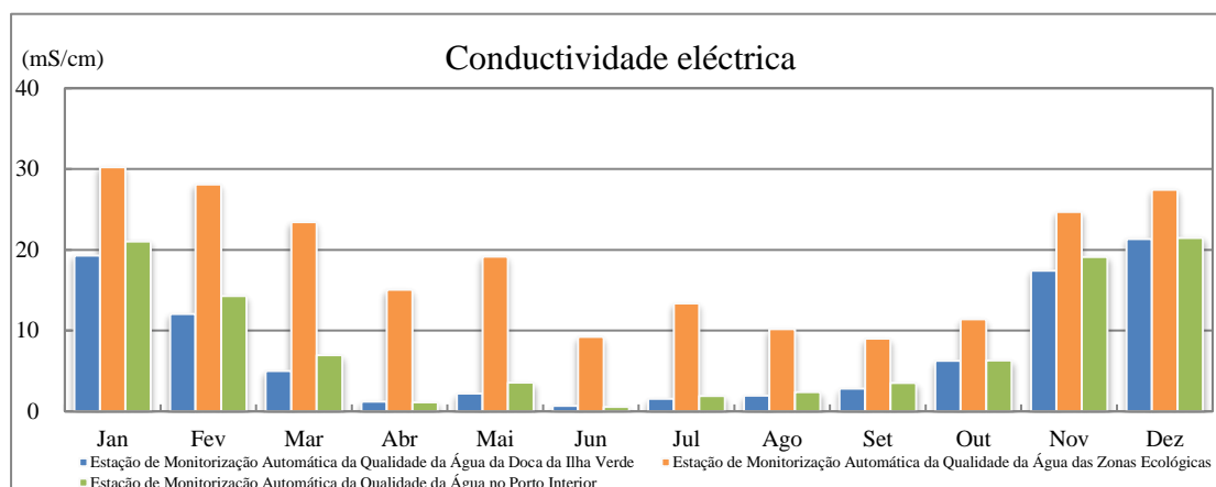
Figura 3.2a Variação da média mensal da condutividade eléctrica registada nas estações de monitorização automática da qualidade da água, em 2020
