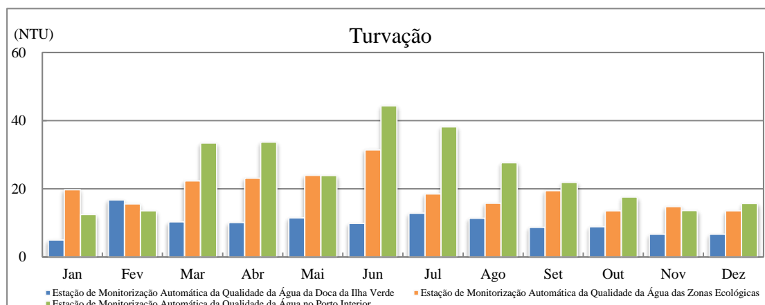
Figura 3.4 Variação da média mensal da turvação registada nas estações de monitorização automática da qualidade da água, em 2020
