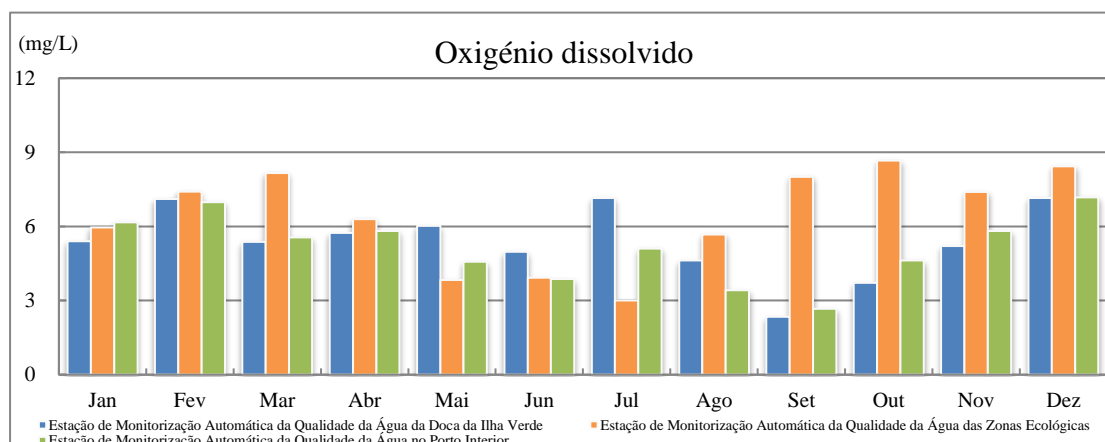
Figura 3.5 Variação da média mensal do oxigénio dissolvido registada nas estações de monitorização automática da qualidade da água, em 2020
