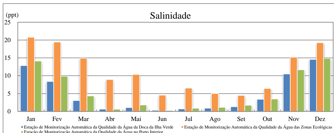
Figura 3.2b Variação da média mensal da salinidade registada nas estações de monitorização automática da qualidade da água, em 2020
