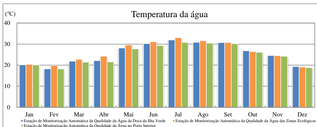
Figura 3.1 Variação da média mensal da temperatura da água registada nas estações de monitorização automática da qualidade da água, em 2020
