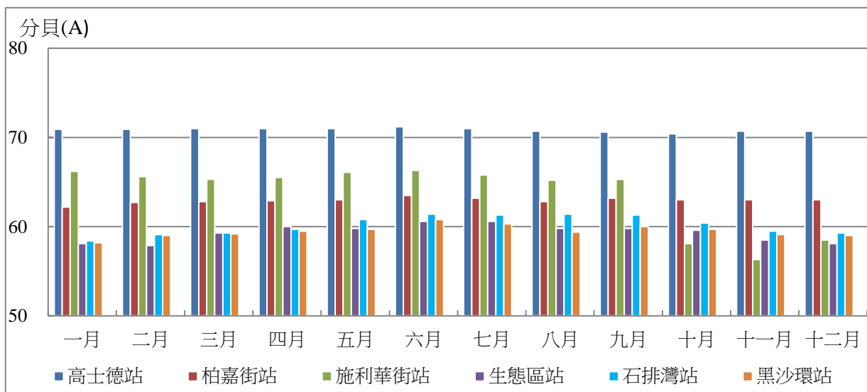
圖 3.3 2021 年各環境噪聲監測站夜間月平均等效連續聲級（ L_{eq} ）變化圖
