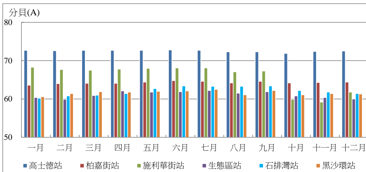
圖 3.4 2021 年各環境噪聲監測站黃昏月平均等效連續聲級 ( L_{eq} ) 變化圖
