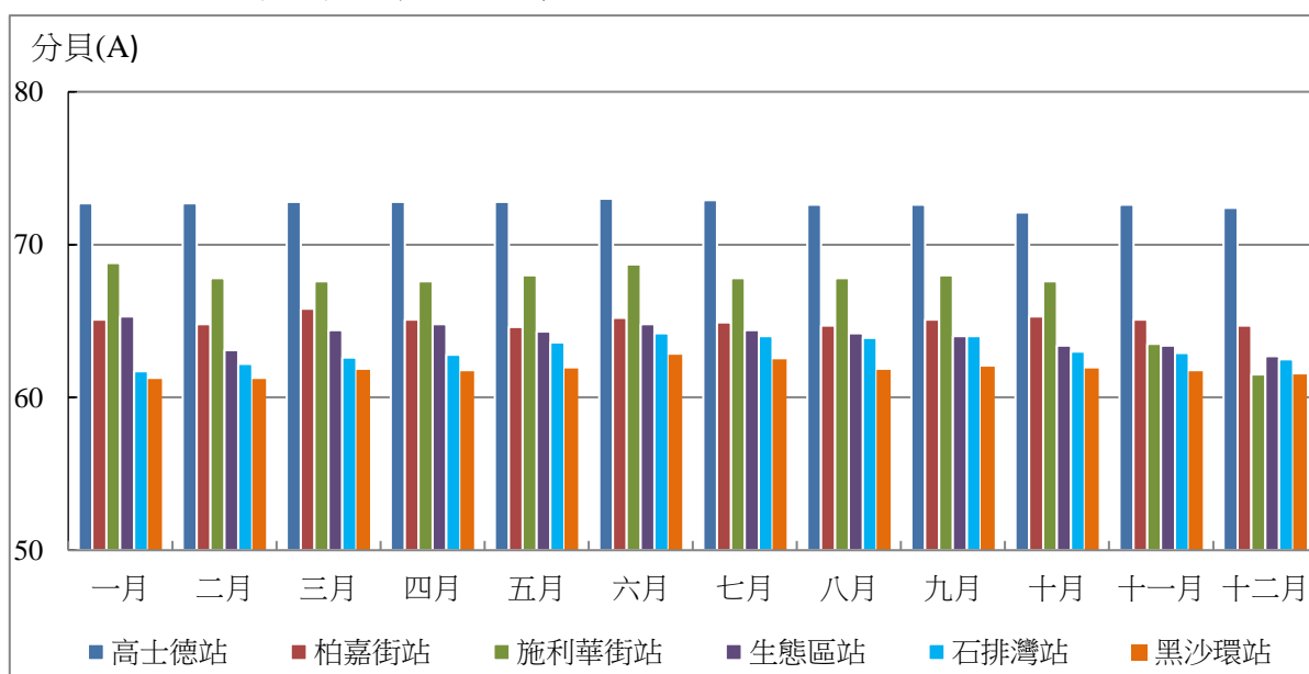
圖 3.1 2021 年各環境噪聲監測站 24 小時月平均等效連續聲級 ( L_{eq} ) 變化圖
