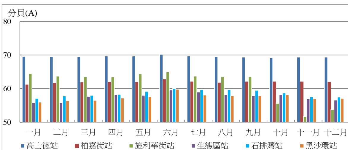
圖 3.5 2021 年各環境噪聲監測站深宵月平均等效連續聲級 ( L_{eq} ) 變化圖
