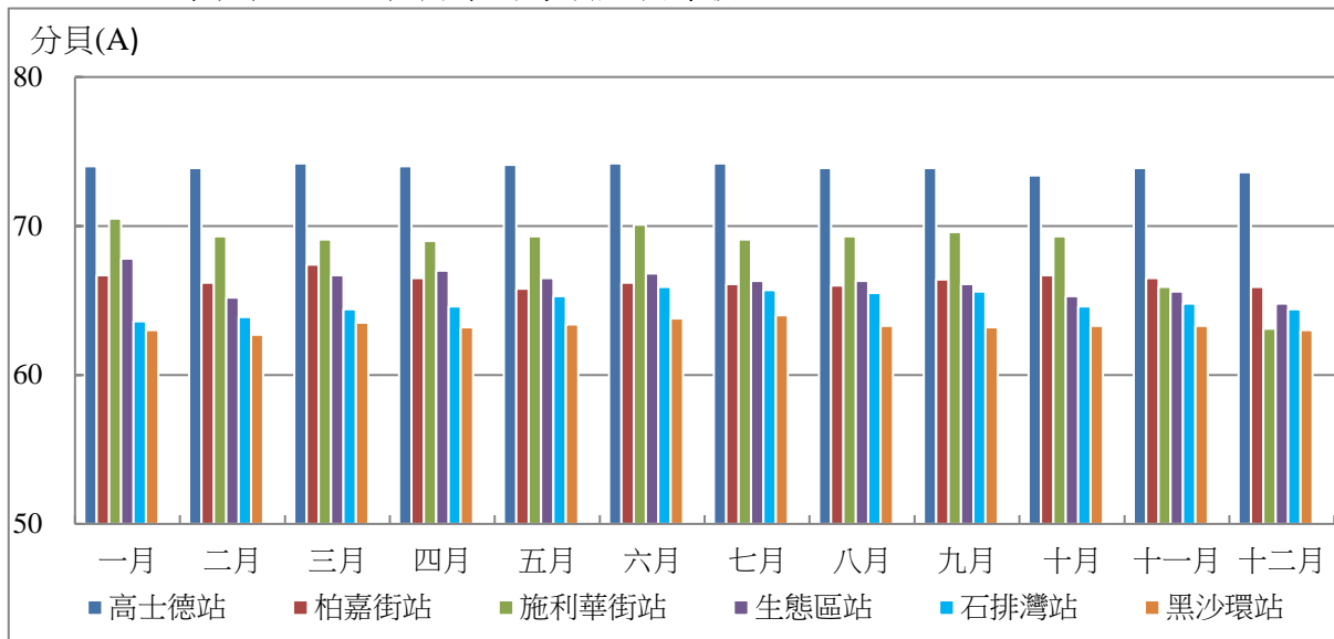
圖 3.2 2021 年各環境噪聲監測站日間月平均等效連續聲級（ L_{eq} ）變化圖
