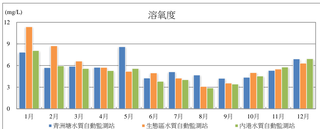
圖 3.5 2021 年各水質自動監測站溶氧度月平均值變化圖
