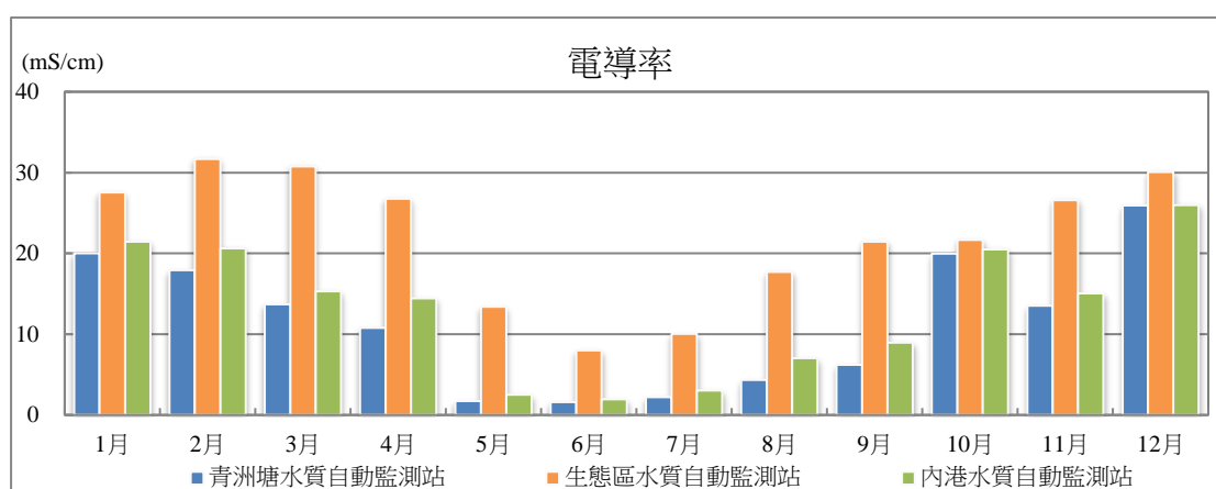
圖 3.2a 2021 年各水質自動監測站電導率月平均值變化圖
