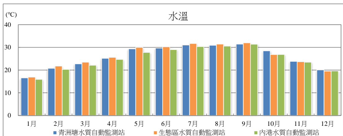
圖 3.1 2021 年各水質自動監測站水溫月平均值變化圖
