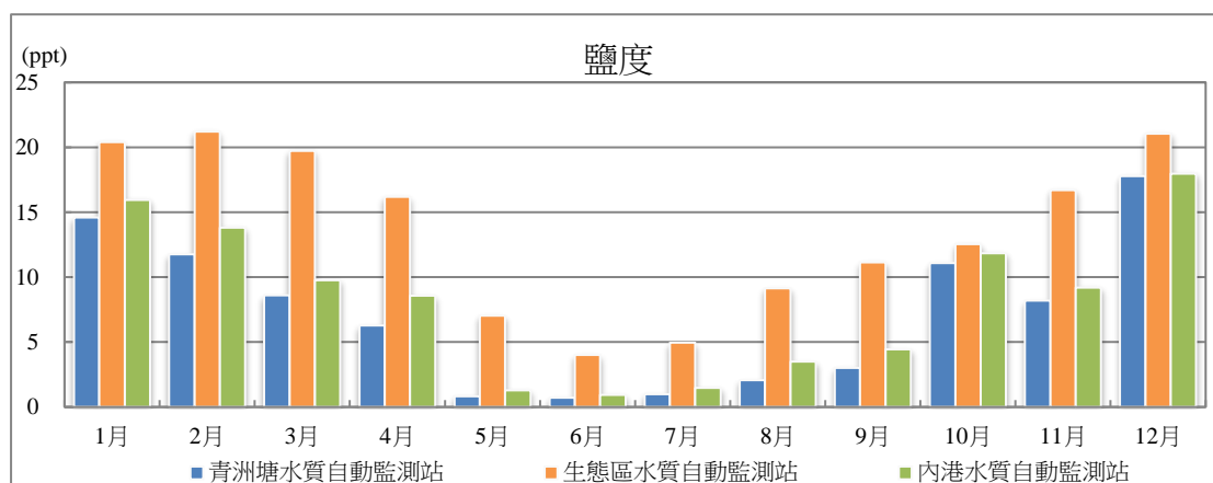
圖 3.2b 2021 年各水質自動監測站鹽度月平均值變化圖
