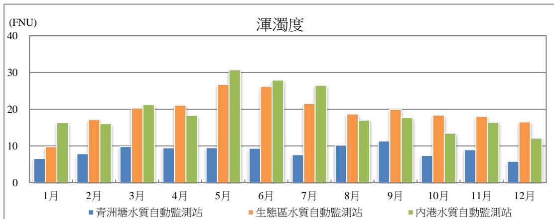
圖 3.4 2021 年各水質自動監測站渾濁度月平均值變化圖
