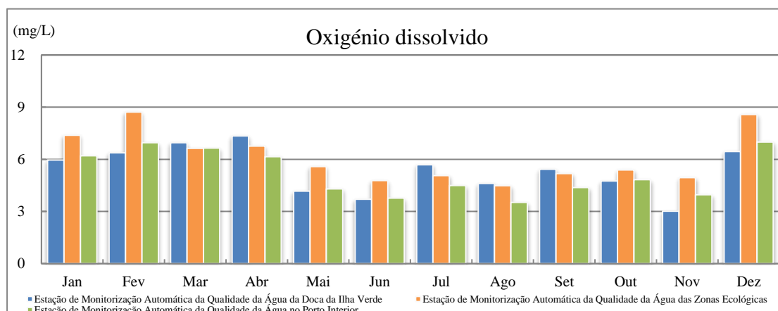
Figura 3.5 Variação da média mensal do oxigénio dissolvido registada nas estações de monitorização automática da qualidade da água, em 2022
