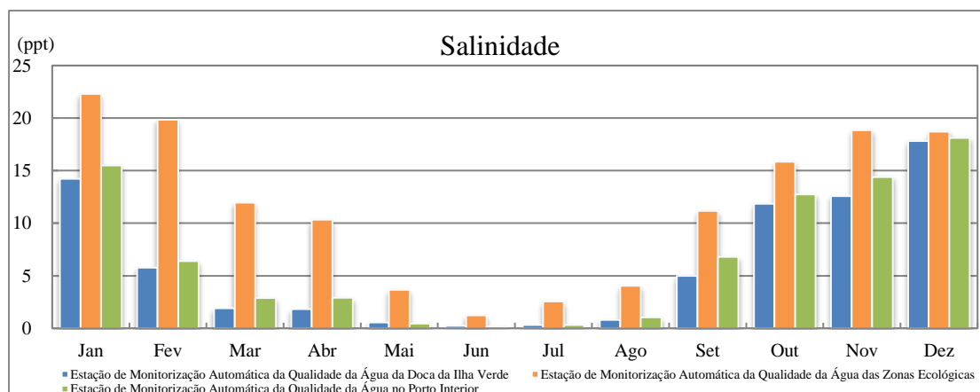
Figura 3.2b Variação da média mensal da salinidade registada nas estações de monitorização automática da qualidade da água, em 2022
