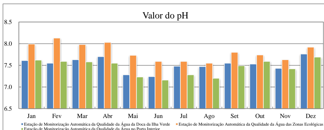
Figura 3.3 Variação da média mensal do valor do pH registada nas estações de monitorização automática da qualidade da água, em 2022
