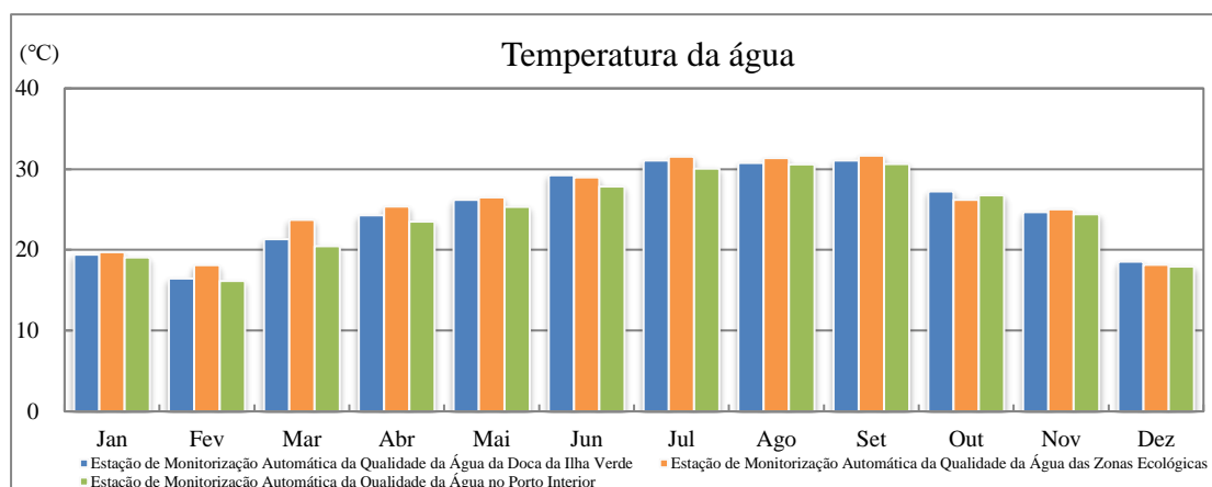
Figura 3.1 Variação da média mensal da temperatura da água registada nas estações de monitorização automática da qualidade da água, em 2022
