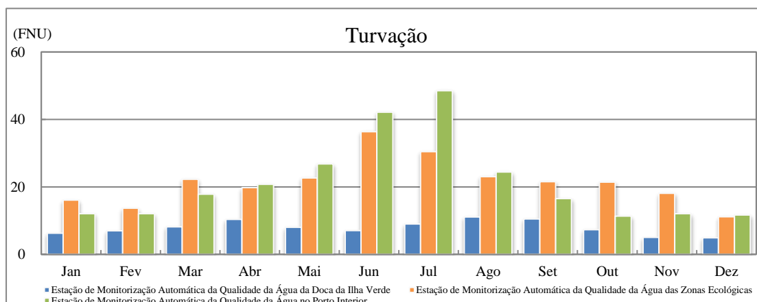
Figura 3.4 Variação da média mensal da turvação registada nas estações de monitorização automática da qualidade da água, em 2022
