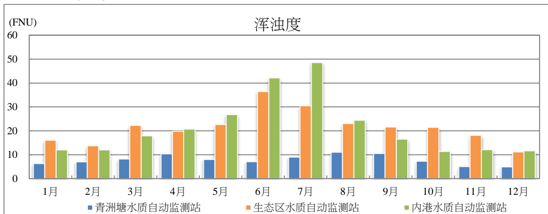
图 3.4 2022 年各水质自动监测站浑浊度月平均值变化图
