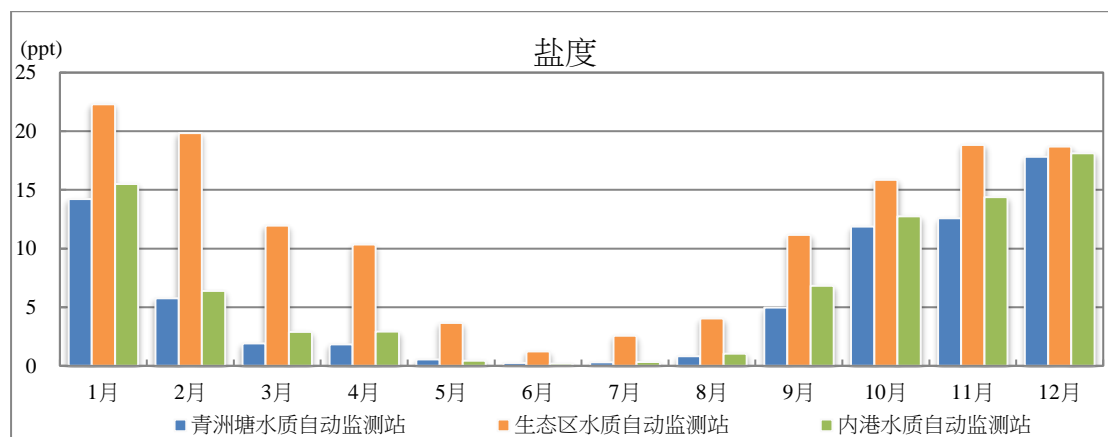
图 3.2b 2022 年各水质自动监测站盐度月平均值变化图
