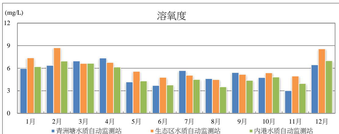
图 3.5 2022 年各水质自动监测站溶氧度月平均值变化图
