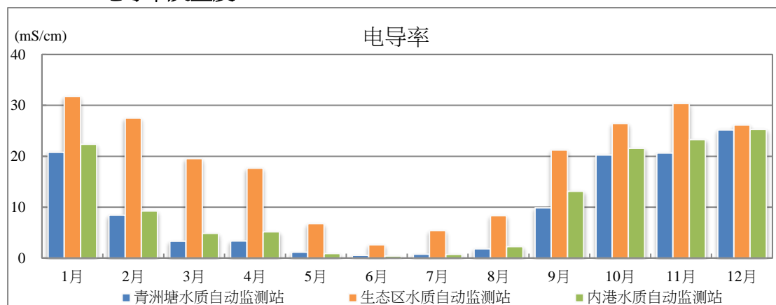
图 3.2a 2022 年各水质自动监测站电导率月平均值变化图
