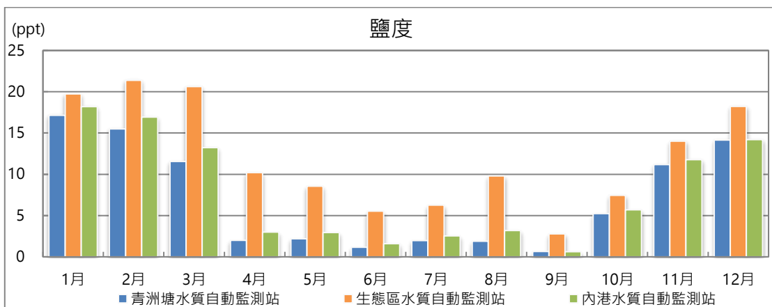
圖 3.2b 2023 年各水質自動監測站鹽度月平均值變化圖
