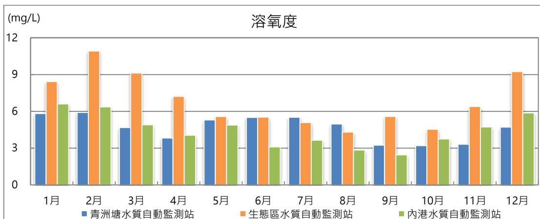
圖 3.5 2023 年各水質自動監測站溶氧度月平均值變化圖
