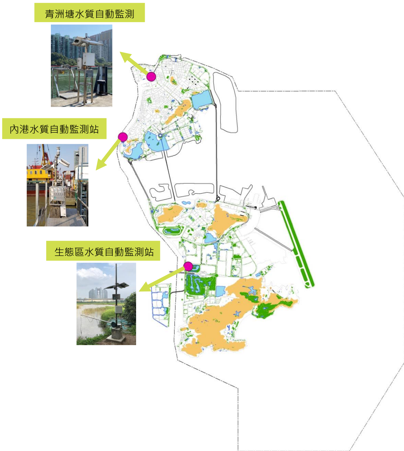
圖 1.1 水質自動監測站位置
