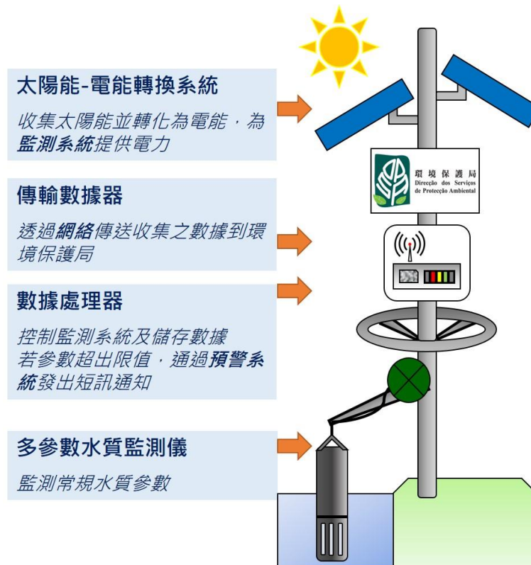
圖 2.1 水質自動監測站儀器組件
