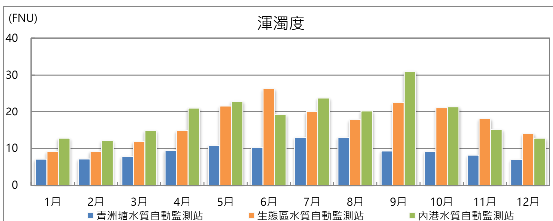
圖 3.4 2023 年各水質自動監測站渾濁度月平均值變化圖
