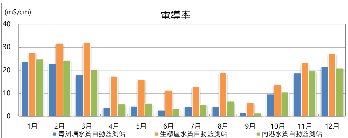
圖 3.2a 2023 年各水質自動監測站電導率月平均值變化圖
