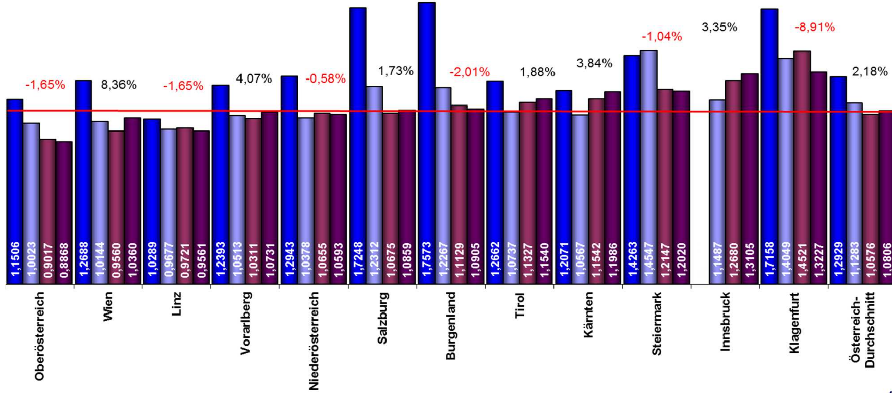
Netznutzungs- und Netzverlustentgelt Netzebene 4 BD = 5.700 h Cent/kWh
