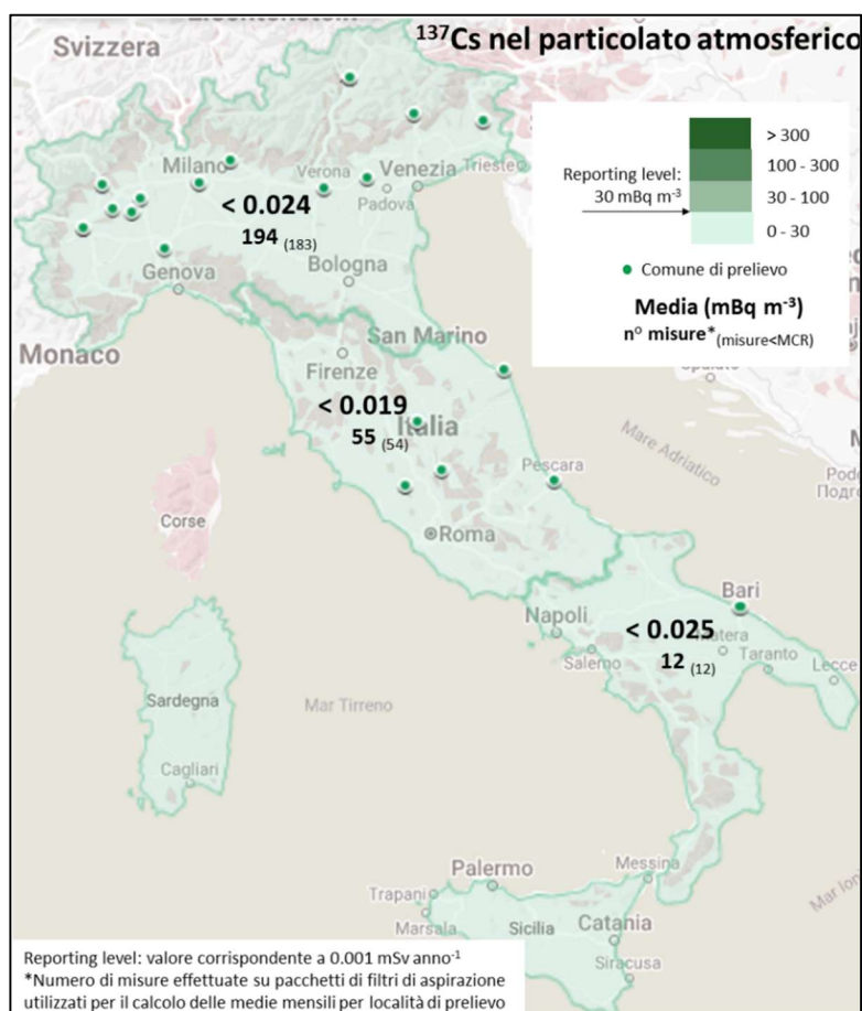
Figura 2 - Media annuale della concentrazione di attività di Cs-137 nel particolato atmosferico
