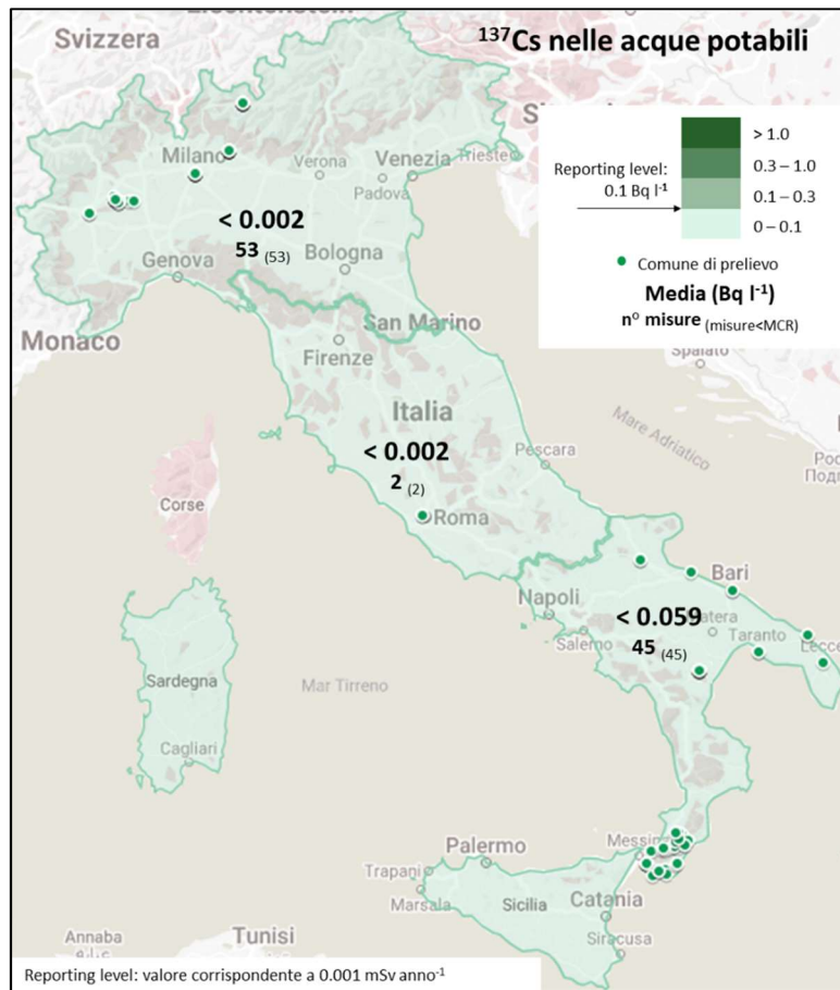
Figura 8 - Media annuale della concentrazione di attività di Cs-137 nelle acque potabili
