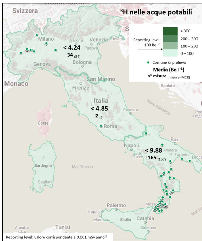
Figura 10 - Media annuale delle concentrazioni di attività di H-3 nelle acque potabili
