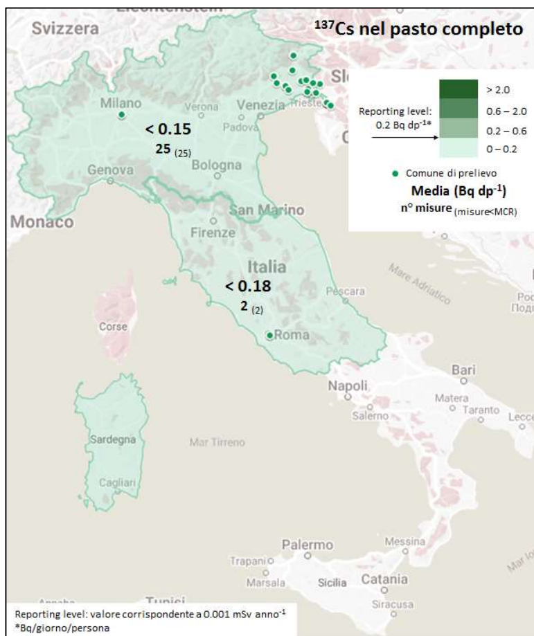
Figura 16 - Concentrazione media annuale di attività di Cs-137 nel pasto completo
