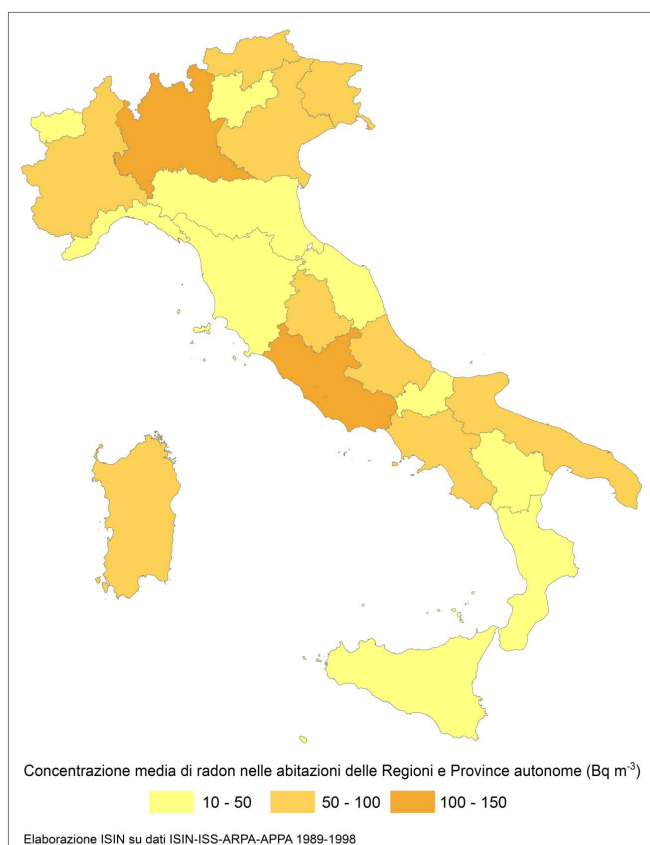
Figura 20 - Carta tematica delle concentrazioni medie di radon stimate dall'indagine nazionale 1989-1998 nelle Regioni e Province autonome
