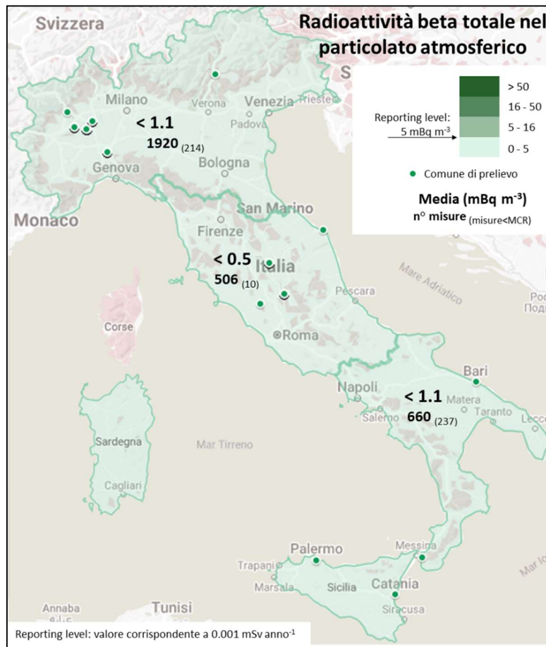
Figura 3 - Media annuale della concentrazione di attività di beta totale nel particolato atmosferico
