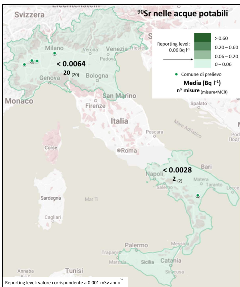
Figura 9 - Media annuale delle concentrazioni di attività di Sr-90 nelle acque potabili
