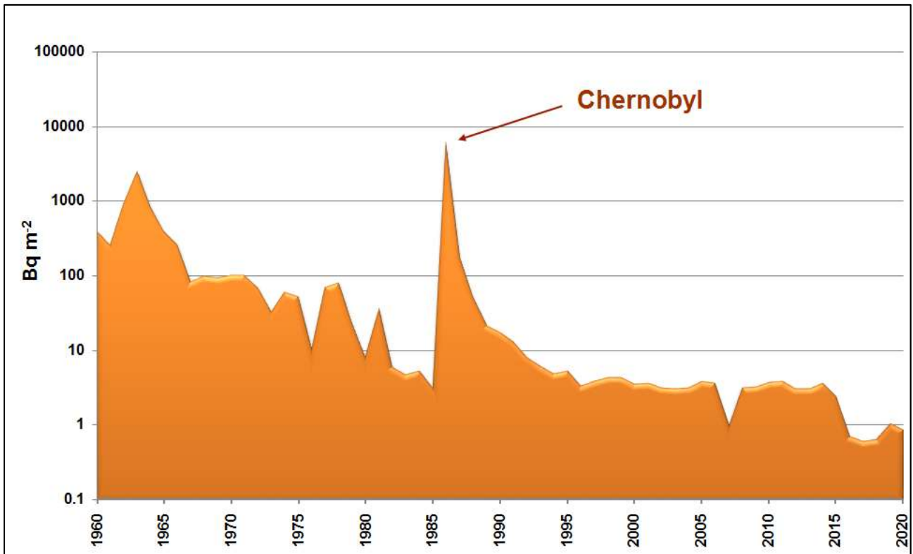
Figura 6 - Andamento della concentrazione di attività di Cs-137 nella deposizione al suolo
