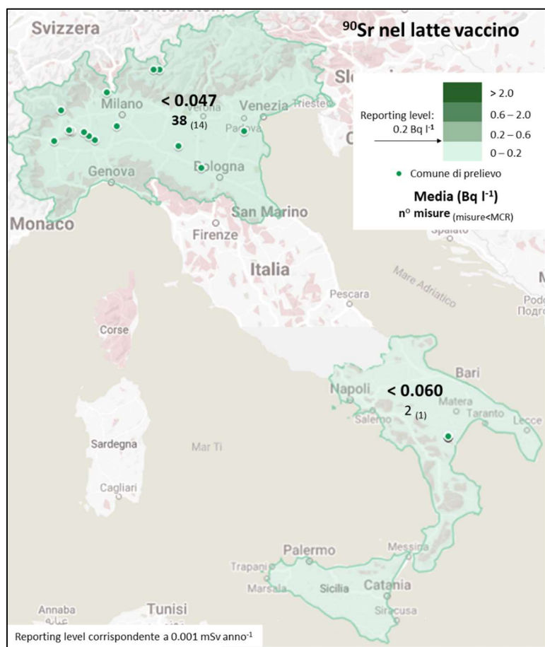
Figura 15 - Concentrazione media annuale di attività di Sr-90 nel latte vaccino
