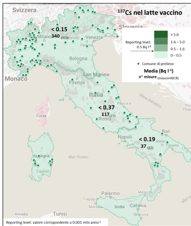
Figura 13 – Media annuale della concentrazione di attività di Cs-137 nel latte vaccino
