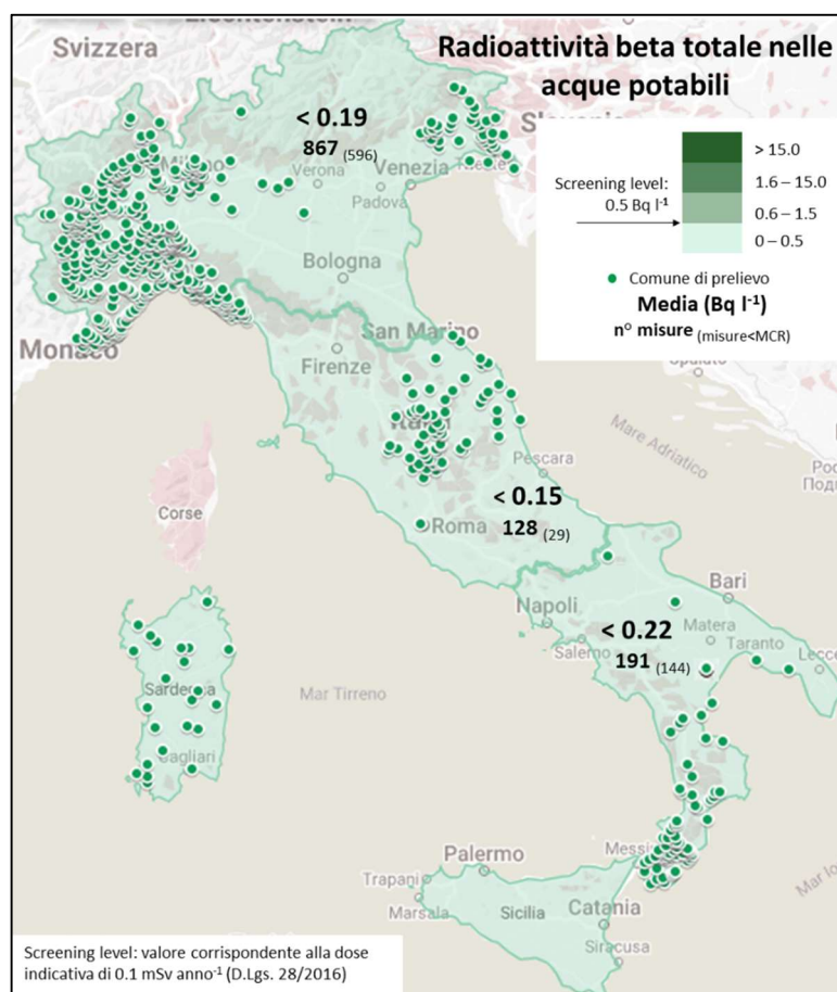
Figura 12 - Media annuale delle concentrazioni di attività beta totale nelle acque potabili
