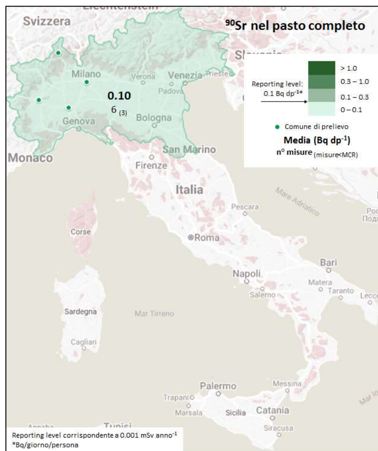
Figura 17 - Media annuale delle concentrazione di attività di Sr-90 nel pasto completo
