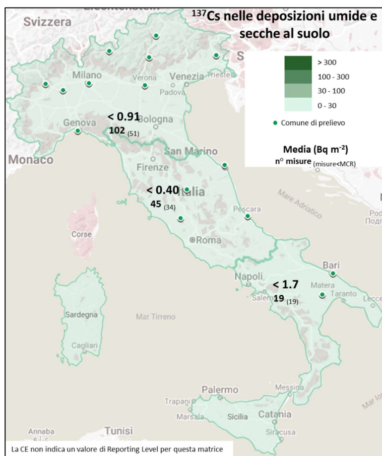
Figura 5 - Concentrazione di attività annuale di Cs-137 nella deposizione al suolo
