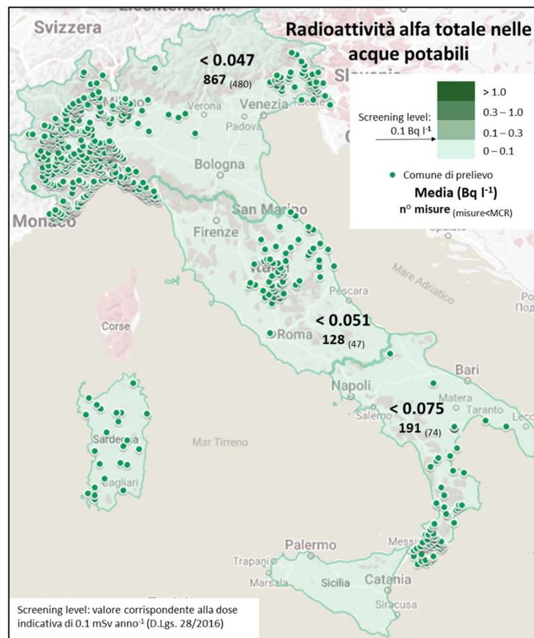
Figura 11 - Media annuale delle concentrazioni di attività alfa totale nelle acque potabili
