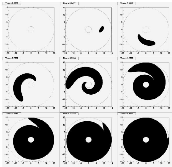
Рис. Численная модель распространения волны панспермии по галактическому диску. Время на рисунке указано в галактических годах. Последовательные времена, соответствующие приведенным фазам эволюции волны, есть (слева направо и сверху вниз): 0.0060, 0.2477, 0.5015, 0.7522, 0.9996, 1.2522, 1.5019, 1.7518, 2.0053. Галактика вращается против часовой стрелки. В качестве начальной точки для волны панспермии выбрано реальное положение Солнца в Галактике (8,5 кпс от центра)
