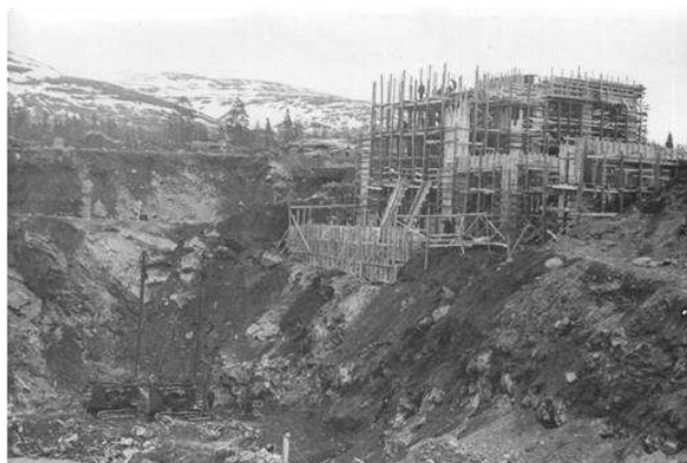
Подготовка котлована для корпуса крупного дробления АНОФ-2. Июнь 1958 г. ГОКУ ГАМО в г. Кировске. Ф. Р-520. Оп. 1. Д. 566.
