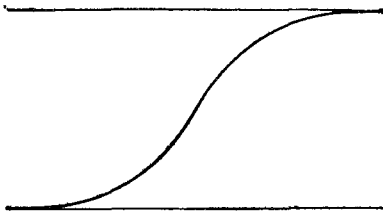
Рис. 45. Логистическая кривая
