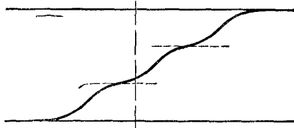
Рис. 46. Многоциклическая логистическая кривая
