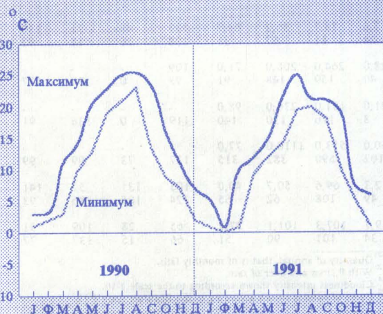
Граф. 1.1. ТЕМПЕРАТУРА ВОДЕ НА ДУНАВУ TEMPERATURE OF THE DENEUBE WATER
