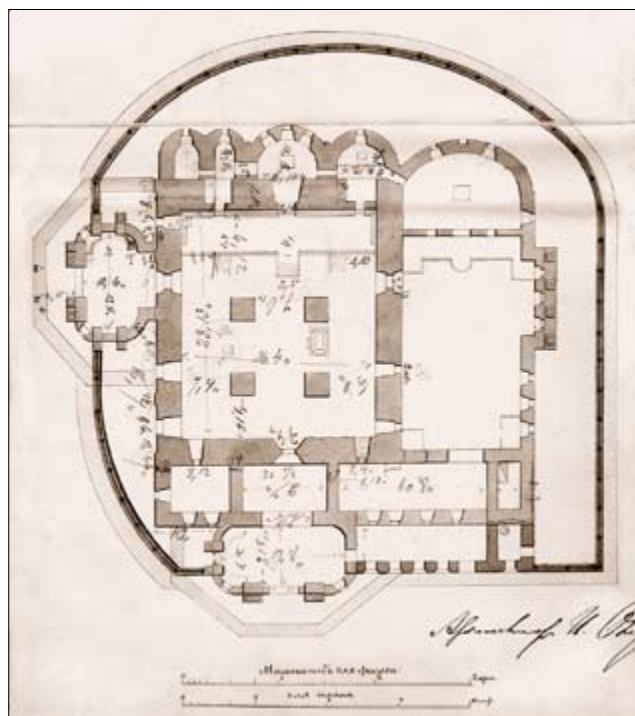
План Успенского собора. Проект сооружения ограды и паперти (не осуществлен). 1881
