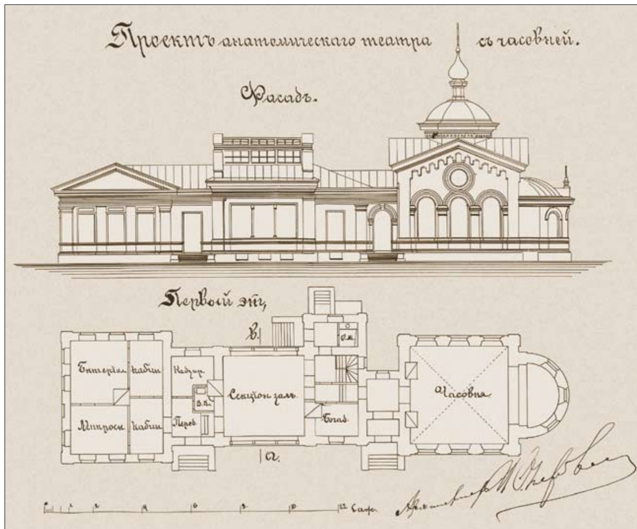
Фасад и план анатомического театра с часовней. 1898
