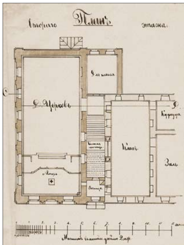
План Покровско-Мариинской церкви. 1885
