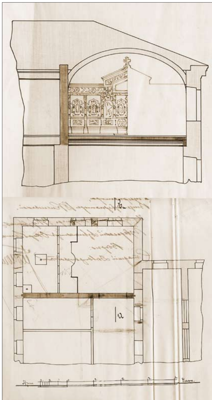
Эскиз иконостаса и план домового храма при губернаторском доме. 1906
