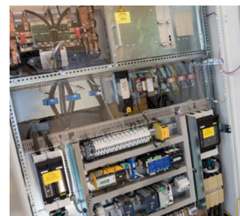
oben: Speicherblock, unten: Steuerung Heimschuh, alle Fotos: Energie Steiermark/Symbol
