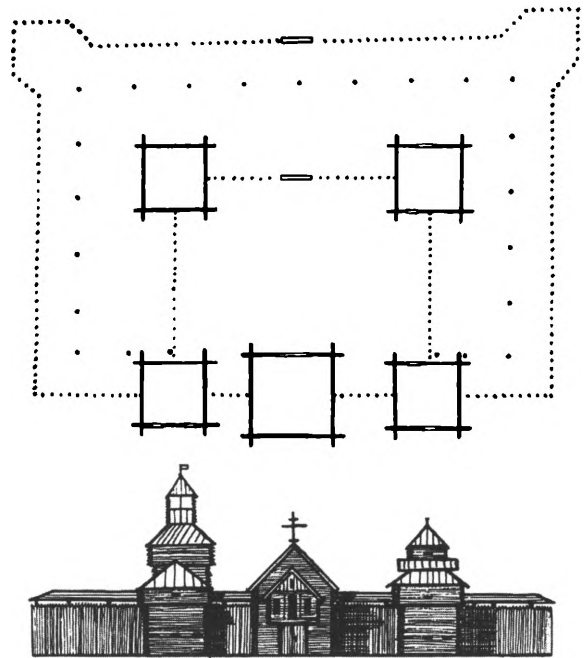
Селенгинский острог в 1669 г. Реконструкция В.И. Кочедамова с исправлениями А.Р. Артемьева
